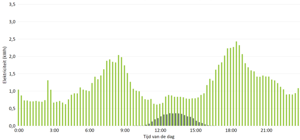
Figuur 21: Melkveehouderijbedrijf met een traditioneel melksysteem (TMS-PV6) met een jaarproductie van 1.300.000 kg melk en een gebruik van \pm 45 kWh/1.000 kg melk. Gemiddelde gebruik en terug levering in de maand december (figuur van 'Uw Agrarisch Bouwadviseur').
