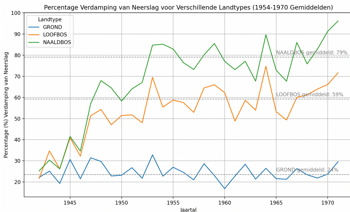
Figuur 10: Resultanten van verdampingsmetingen in Castricum periode 1956-1969 (bron: Van der Molen, 1975), Lysimeters Wageningen in de periode 1952 tot 1965. De Gruyter (1957) heeft metingen uitgevoerd in 1942 tot 1945. De verdamping van neerslag is voor dit rapport uitgedrukt als percentage van de totale neerslag in dat jaar. De gemiddelde lijn is bepaald op de periode 1950 tot 1970. Verdamping vanaf de grond is gemiddeld 24%.
