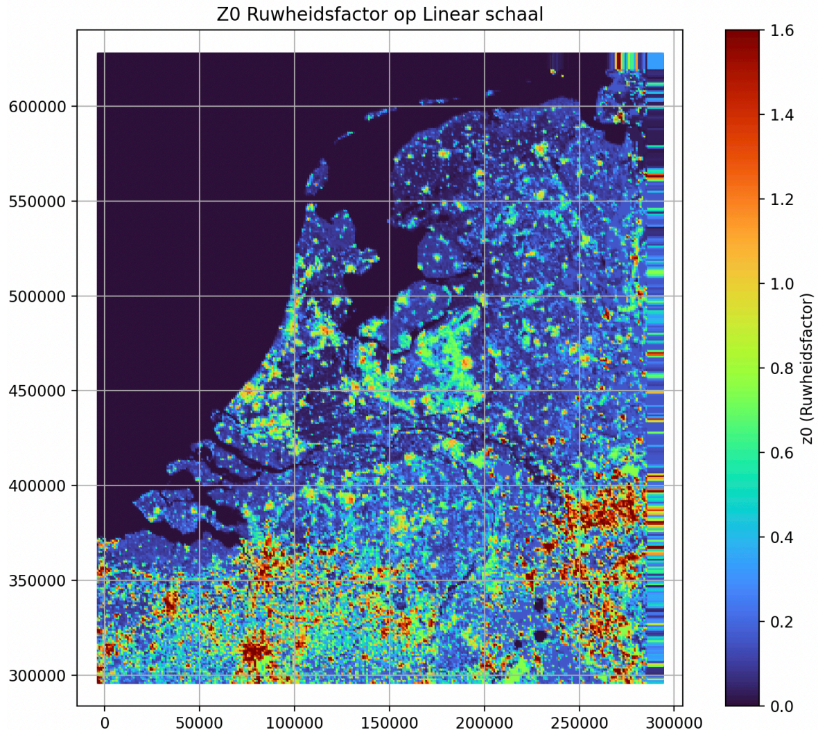
Figuur 2 – Ruwheidskaart van Nederland. De ruwheid van de steden valt erg op. Bron: Landelijk Grondgebruik Nederland (LGN7). Volgens de theorie betekent meer ruwheid een lagere weerstand R_a en R_b , waardoor de depositiesnelheid hoger kan zijn. Uiteindelijk wordt R_{\text{totaal}} immers ook bepaald door de waarde van R_c .
