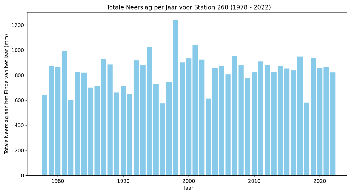
Figuur 7: Neerslag op station 260 (De Bilt) duidelijk zijn de drogere en nattere periode te zien die goed correleren met de pieken en dalen zoals deze in de Figuren 5 en 7 zichtbaar zijn.
