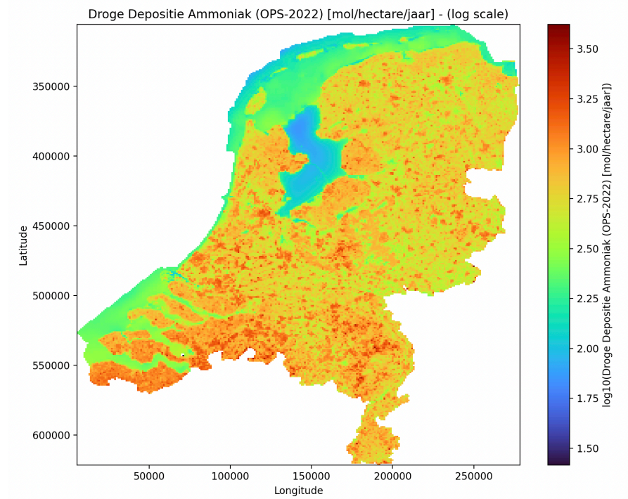
Figuur 11a: berekende droge NH 3 depositie per vierkante kilometer en uitgedrukt in mol per hectare per jaar en afgedrukt op een logaritmische schaal. Deze dataset is gegenereerd met OPS 2022.
