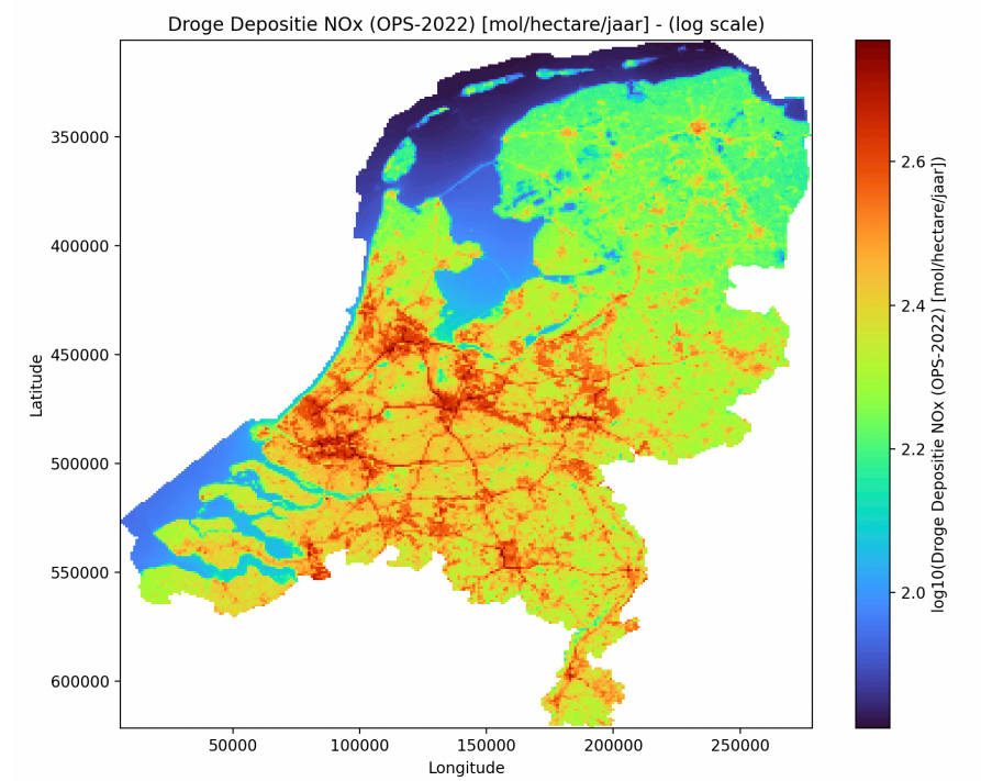
Figuur 11b: berekende droge NO x depositie per vierkante kilometer en uitgedrukt in mol per hectare per jaar en afgedrukt op een logaritmische schaal. Deze dataset is gegenereerd met OPS 2022.
