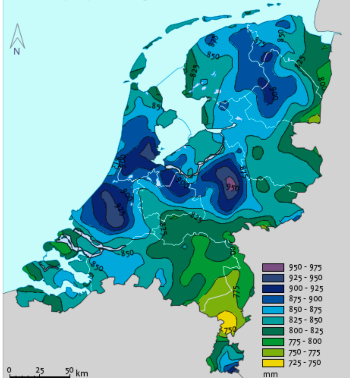
Figuur 5: Gemiddelde jaarlijkse hoeveelheid neerslag in Nederland van 1981 tot 2010 (bron www.klimaatatlas.nl ). Het is niet bekend of deze neerslag verdeling anno 2024 anders is dan vijftien jaar geleden het geval was. Ook is de hypothese dat de werkelijke natte depositie vooral afhangt van de (hevigheid) van de lokale neerslag in combinatie met de hoogte van de ammoniakconcentratie.
