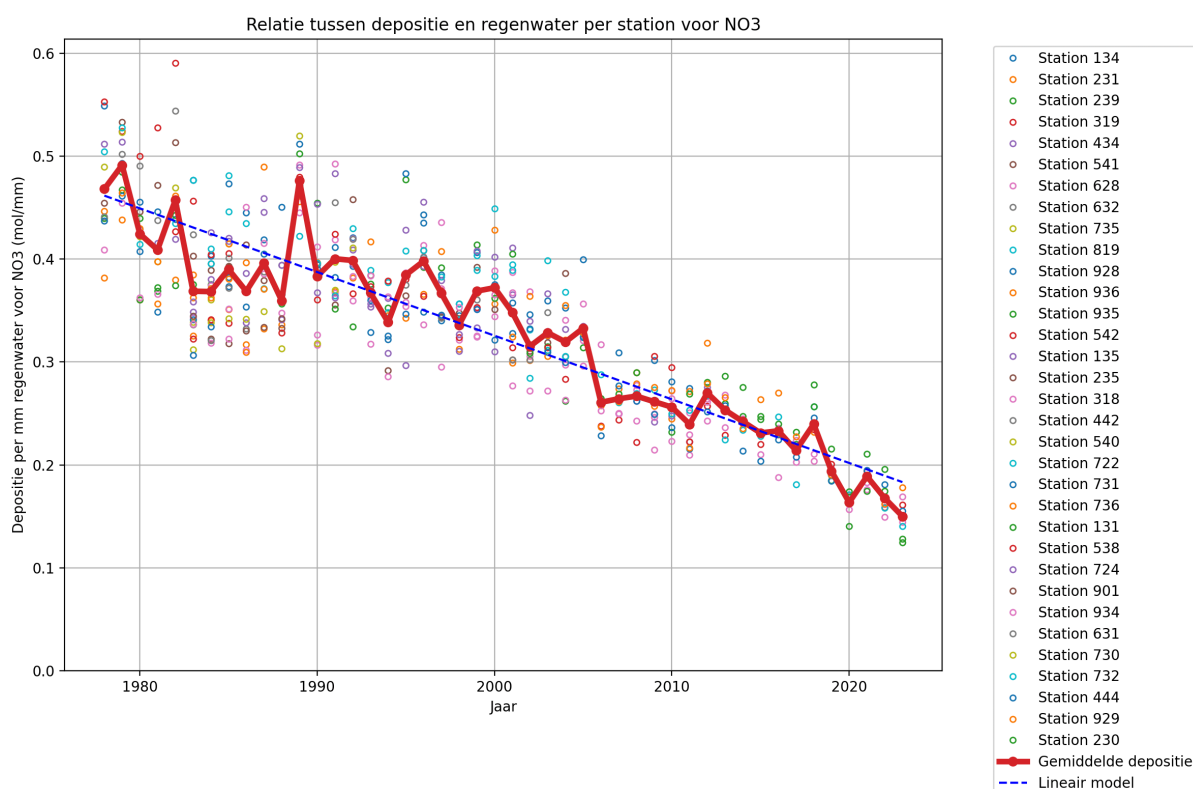
Figuur 8: De natte depositie data van alle stations is gedeeld door de werkelijke regenval op dat station in dat jaar om tot een depositie per millimeter regenwater te komen. Deze parameter kan gezien worden als een jaarlijkse concentratie term en daarmee een indicator voor 'de kwaliteit' van de lucht in dat jaar. De meeste pieken en dalen die sterk afwijken van het (arbitrair) gekozen lineaire model zijn te verklaren doordat er in het betreffende jaar sprake was van extreme droogte of juist natheid. We zien dat de stikstofoxide (NOx) deken boven Nederland met ongeveer 60% is gedaald.
