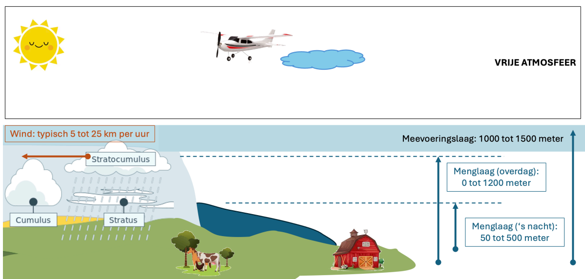
Figuur 4: De verspreiding van ammoniak en stikstofoxiden en grafische toelichting op de menglaag.
