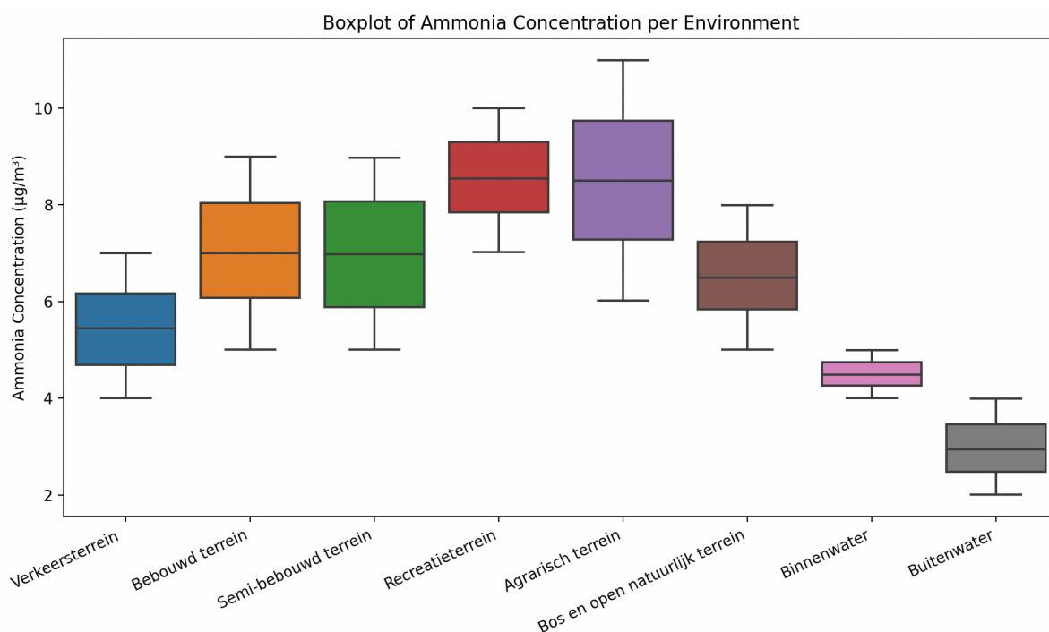
Figuur 10: Boxplot van de ammoniakconcentratie inschattingen op basis van de GCN kaart 2022. We hebben een lineaire verdeling verondersteld in het model. Minimale en maximale waarde staan in Tabel 9. Resultaat van de Monte Carlo simulatie N=500. Zie ook Figuur 11 t.a.v. de concentratievoorspellingen over heel Nederland.
