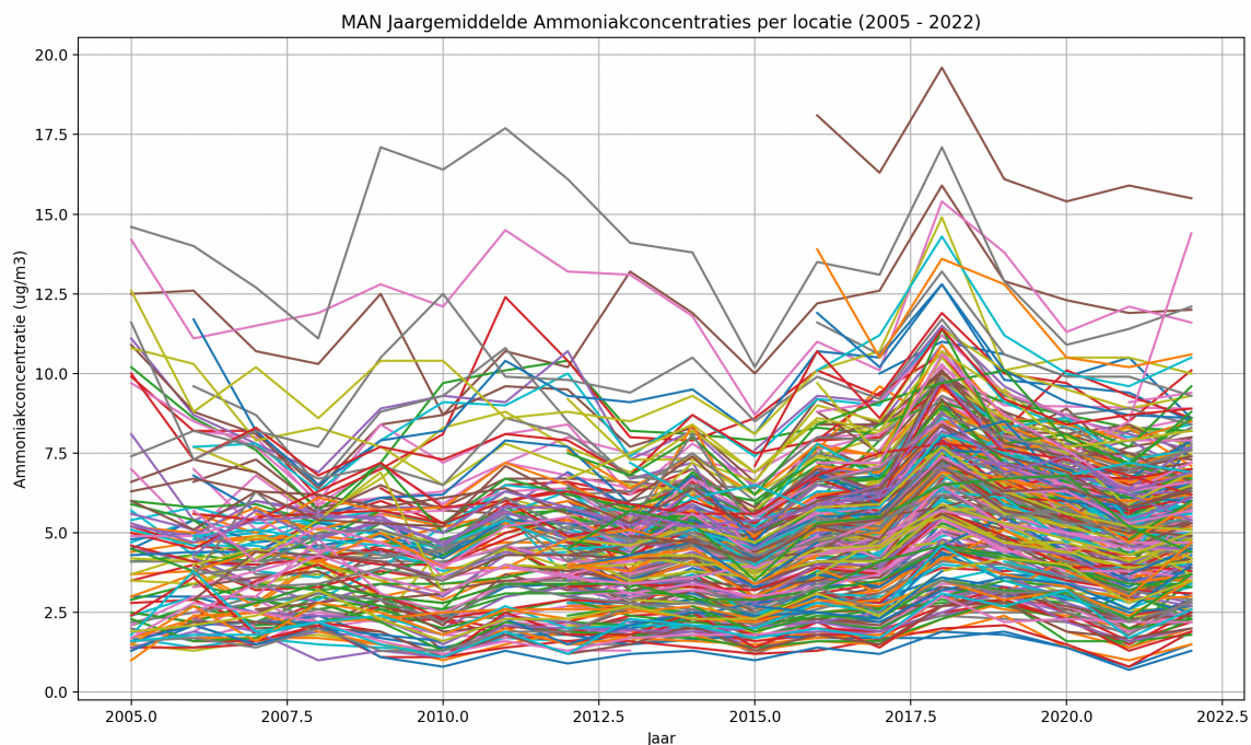
Figuur 1: De jaargemiddelde MAN ammoniakconcentratie per meetpunt. Deze grafiek is nogal “druk” en alleen hier weergegeven om een globale indruk te geven van de hoeveelheid data die beschikbaar is om statistische verwerking uit te voeren. Vanaf 2012 zijn er meer meetlocaties gecreëerd. Bewust is de legenda met daarin de namen van de meetlocaties niet opgenomen, deze legenda lijst zou veel te lang zijn daar er immers 110 MAN gebieden zijn en de leesbaarheid niet vergroten. Opvallend is de verhoging in het jaar 2018.
