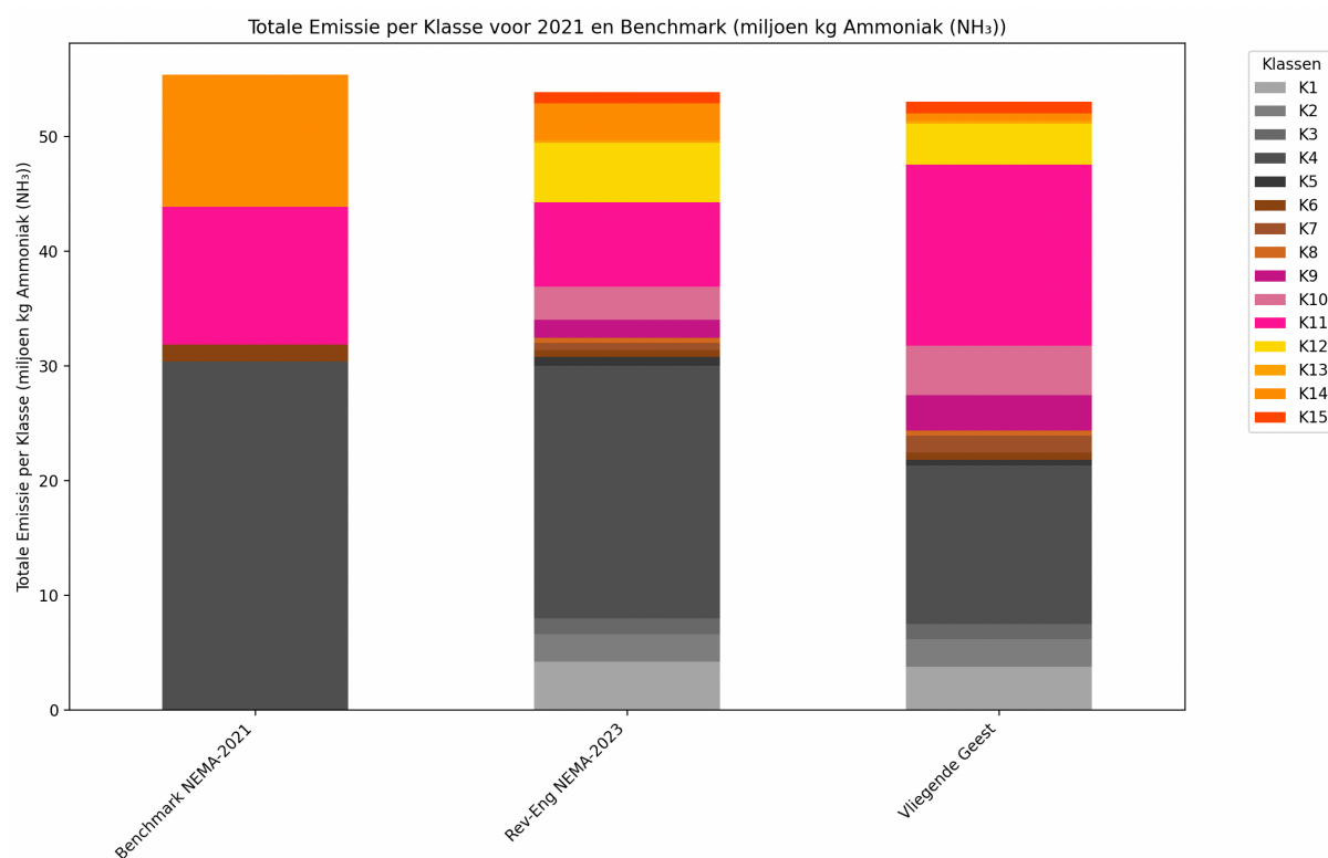
Figuur 6: Ammoniakemissie uitgedrukt in miljoen kilogram ammoniak voor het jaar 2021.
