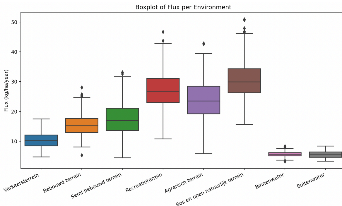
Figuur 11: Boxplot van de berekende droge depositie in kilogram ammoniak per hectare per jaar. De depositie is berekend door de ammoniak concentratie te vermenigvuldigen met de depositie-snelheid. Resultaat van de Monte Carlo simulatie N=500
