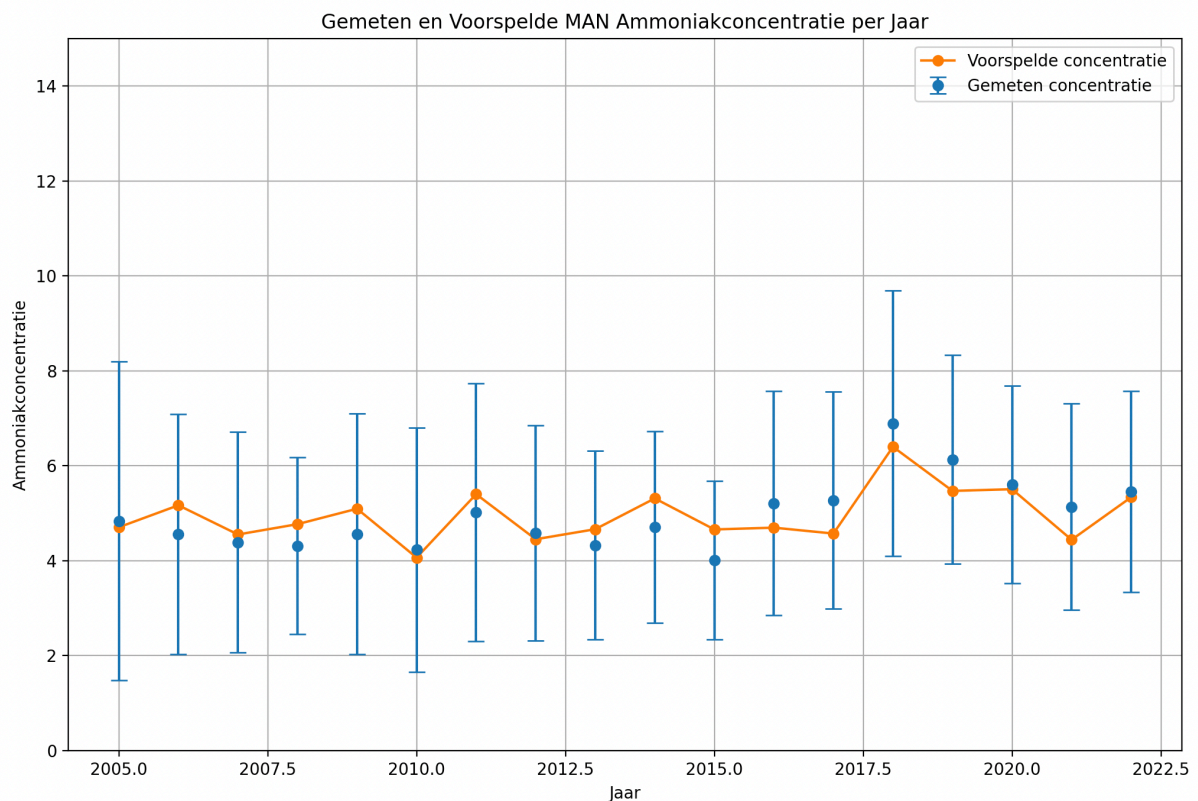
Figuur 5: de gemeten en voorspelde gemiddelde MAN ammoniakconcentratie per jaar. De voorspelde ammoniakconcentratie wordt vooral beïnvloed door de neerslag en de gemiddelde jaartemperatuur. De piek in het aantal runderen in 2016 met een afname van bijna 15% in de jaren erna is niet waar te nemen in de correlatie.
