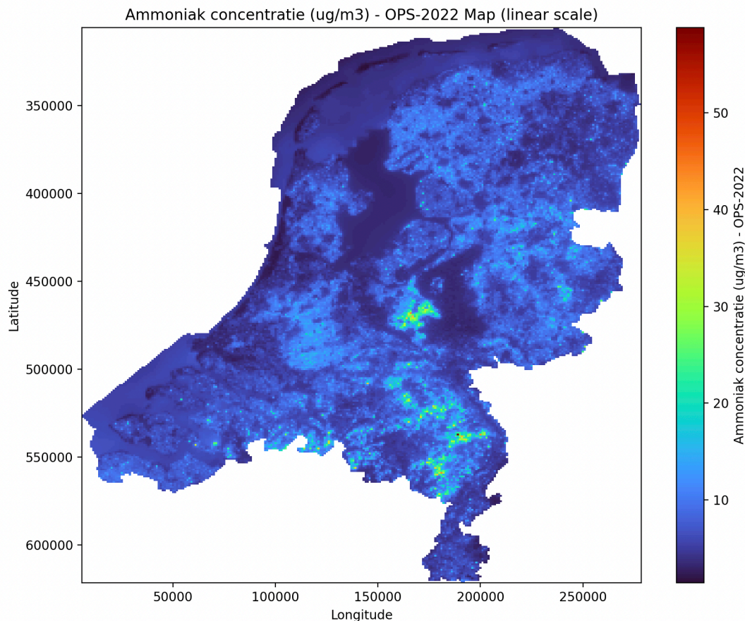
Figuur 6a: De berekende concentratie heatmap (OPS-2022) van de ammoniak concentratie uitgedrukt in \mu\text{g}/\text{m}^3 op een 1 x 1 km grid over Nederland. Duidelijk valt op de hoge ammoniakconcentraties boven de Gelderse Vallei, Noord Limburg en Oost Brabant (de Peel). Boven de Noordzee kust, de Wadden, het IJsselmeer en de Veluwe zijn de berekende concentraties laag. Waarom de concentraties boven de Waddenzee hoger zijn dan boven het IJsselmeer dient nader onderzocht te worden.
