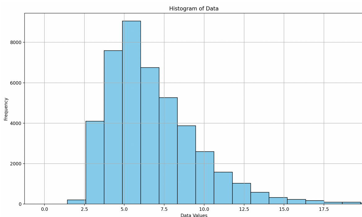
Figuur 11: Histogram van de berekende ammoniakconcentratie boven Nederland. Data uit de OPS-2022 GCN kaart die door RIVM is verstrekt is hiervoor gebruikt. De gemiddelde concentratie op basis van deze OPS berekening is 6,91 \mu\text{g}/\text{m}^3 , en de mediane waarde 6,17 \mu\text{g}/\text{m}^3 . De standaarddeviatie is 3,23 \mu\text{g}/\text{m}^3 . Ter vergelijking: de gemiddelde ammoniakconcentratie bij MAN (Figuur 2) is 5,11 \mu\text{g}/\text{m}^3 (stdev 2,4) en daarmee weer lager dan de gemiddelde ammoniakconcentratie van 7,92 \mu\text{g}/\text{m}^3 voor de LML stations (Figuur 9) in het jaar 2023 (stdev 12,13). LML wordt beïnvloed door voorkomende pieken.
