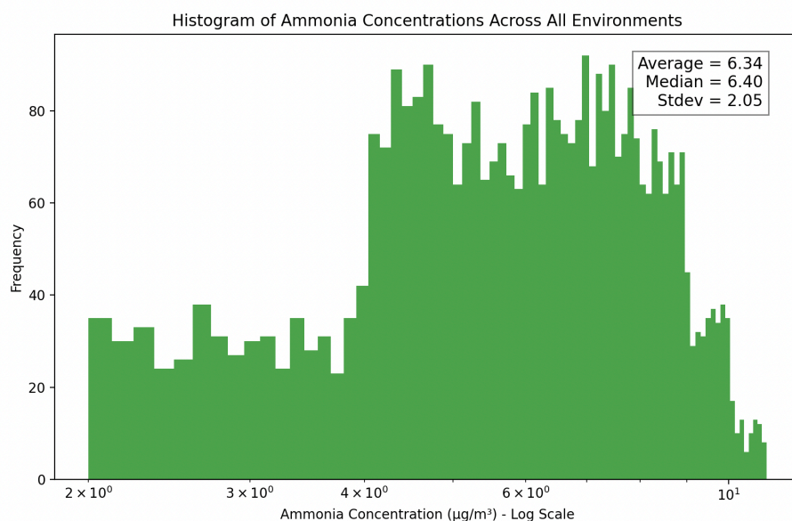
Figuur 12: Histogram van de ammoniak concentratie boven Nederland, resultaat via de Monte Carlo simulatie N=500/ Gemiddelde is iets lager dan de gemiddelde OPS-concentratie, de mediaan is echter net iets hoger dan OPS. Aangezien we de concentratie hebben afgekap op 11 \mu\text{g}/\text{m}^3 is de maximale waarde flink lager dan OPS-2022.
