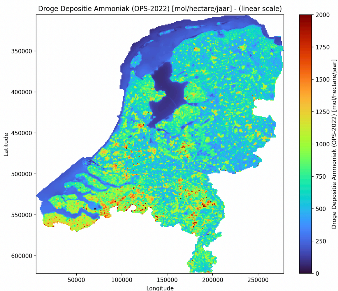
Figuur 8a: berekende droge ammoniak depositie per vierkante kilometer en uitgedrukt in mol per hectare per jaar. De dataset is gegenereerd met OPS 2022. De schaalverdeling is lineair en afgetoet op 2000 mol (er zijn enkele plekken in Nederland waar deze nog hoger is). De intensieve veehouderij gebieden zijn duidelijk zichtbaar. Maar ook erg opvallend is de lage depositie boven water zoals de Oostvaardersplassen en randmeren en opvallend is de hoge depositie boven de (grote) steden die duidelijk 'rood' oplichten. Volgens de gangbare theorie is dat te verklaren door de hogere ruwheid.
