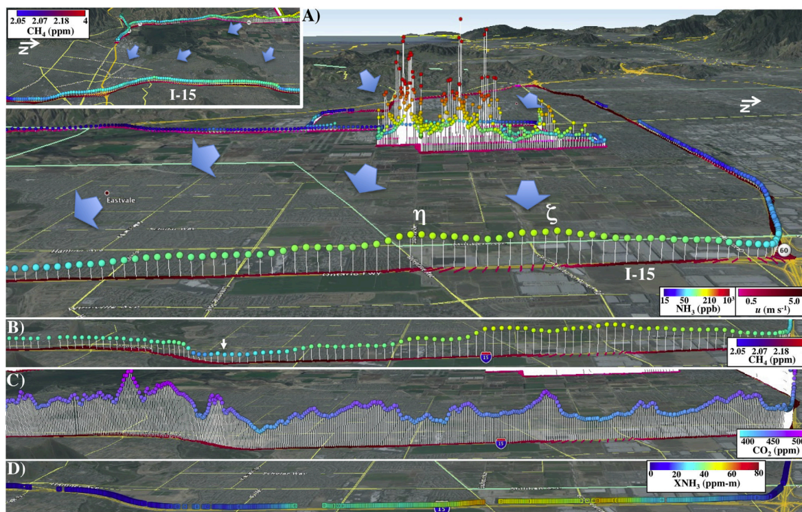
Figuur 14 - Uit Leifer et.al. (2018) A) In situ ammoniak ( \text{NH}_3 ) en windsnelheid ( u ) in de windrichting van het Chino Dairy Complex voor 25 juni 2015. Pijlen geven algemene windpatronen weer. Pieken van pluimen gebruikt in het Gaussische inversiemodel gelabeld ( z , h ). Inzet. Methaan ( \text{CH}_4 ) ten zuiden van Chino en pijlen die de luchtstroom in het veld illustreren. Noordrand van inzetgegevens komt overeen met witte pijl in paneel B. B) In situ \text{CH}_4 , zelfde weergave als in paneel A. C) In situ koolstofdioxide ( \text{CO}_2 ) op het I-15 transect, zelfde weergave als in paneel A. D) MISTIR kolom \text{NH}_3 ( \text{N-NH}_3 ) op het I-15 transect, zelfde weergave als in paneel A. Getoond in de Google Earth-omgeving.
