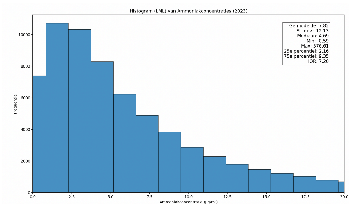
Figuur 9: Histogram van alle beschikbare LML data voor het jaar 2023. Er zijn geen stations uitgesloten waardoor duidelijk wordt hoe de enorme 'pieken' uit Figuur 8 doorwerken in de gemiddelde gemeten waarde van de LML stations. Beter is het om te kijken naar de mediaan. De mediaan ligt op een gematigde maar tevens ook reële 4,69 \mu\text{g}/\text{m}^3 . Dit histogram kan vergeleken worden met het histogram van het MAN netwerk dat in Figuur 2 staat. De gemiddelde ammoniakconcentratie bij MAN is 5,11 \mu\text{g}/\text{m}^3 (stdev 2,4) en dus veel lager dan de hier berekende 7,92 \mu\text{g}/\text{m}^3 (stdev 12,13).
