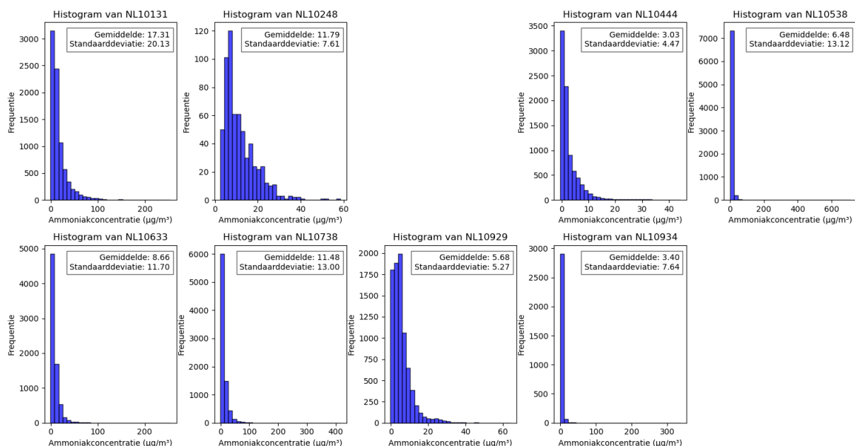
Figuur 10: Histogrammen van de gemeten ammoniakconcentratie boven Nederland in 2022 bij de acht LML locaties. Gemiddelde en standaarddeviatie (µg/m³) staat weergegeven en zijn in tabel 1 vergeleken met de met OPS berekende concentratie. Vijf van de acht stations meten een lagere concentratie dan de voorspelling. Op drie locaties is de voorspelling ongeveer gelijk aan LML.
