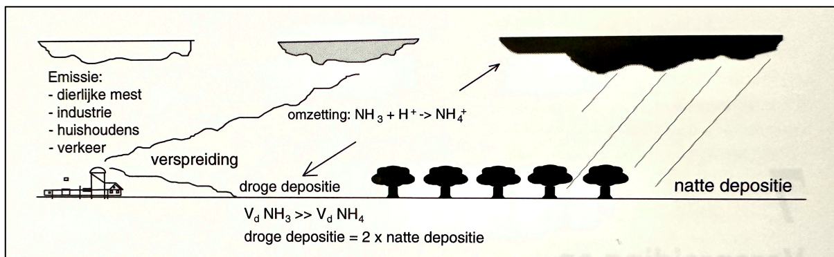
Figuur 1: de emissie, verspreiding, omzetting van ammoniak en de droge en natte depositie. Het ammoniak dossier is relatief gemakkelijk in een plaatje te tonen, de onderliggende chemische, fysische en biologische processen zijn complex. Vooral de depositiewetenschap is relatief jong en nog niet alle aspecten zijn voldoende begrepen c.q. fundamenteel onderzocht.
