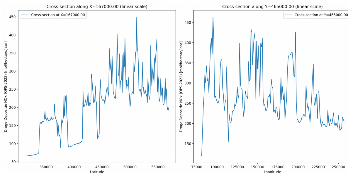
Figuur 9b: Doorsnede Noord-Zuid (links) en Oost-West (rechts). Let op! De y-schaal is niet hetzelfde.
