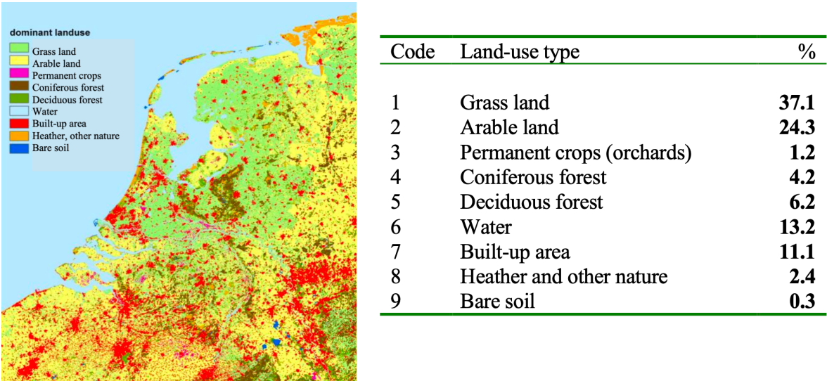
Figuur 12: Nederland verdeeld over de 9 land-use type uit DEPAC (links) en uitgedrukt in oppervlak (rechts), data RIVM.
