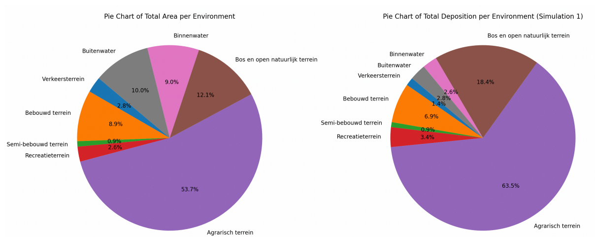
Figuur 15: Verdeling landgebruik Nederland (links) en de verwachte droge depositie verdeling (Resultaat van een Monte Carlo simulatie N=500). Uit Figuur 13 kunnen we echter opmaken dat de verdeling niet zo precies is als deze cirkeldiagram doet suggereren aangezien de onnauwkeurigheid groot is.
