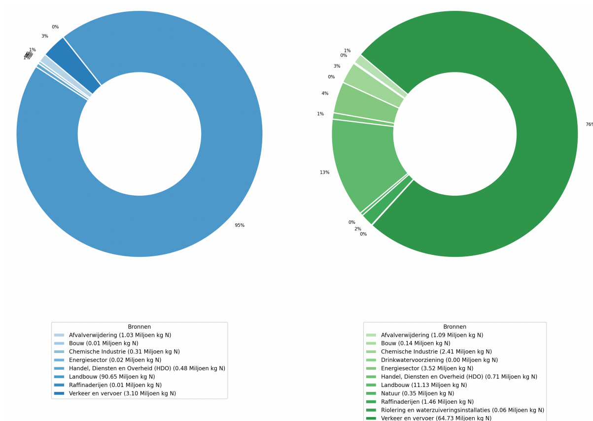
Figuur 4: diagram met percentages over het jaar 2022. De blauwe donut (links) gaat over ammoniak, en de groene donut (rechts) over de stikstofoxiden. Totaal 181,2 miljoen kilogram stikstof. De ammoniakemissies zijn totaal 95,6 miljoen kilo (53%), en de stikstofoxiden totaal 85,6 miljoen kilogram (47%).
