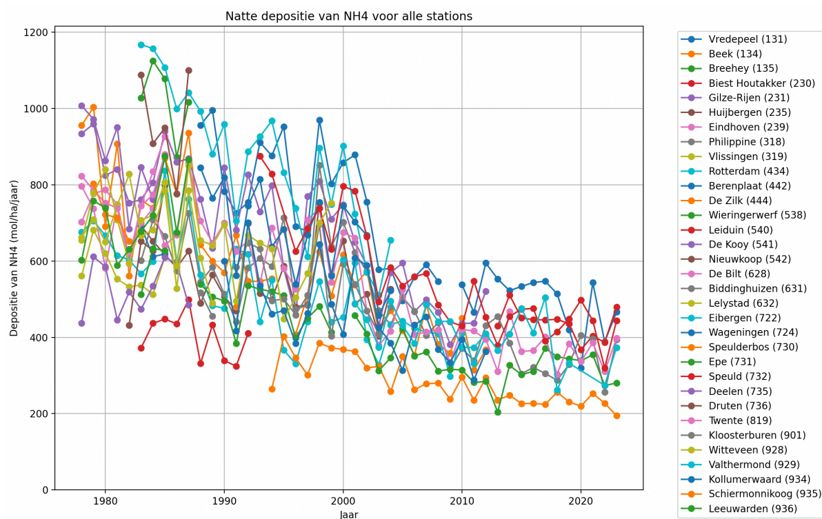
Figuur 1: alle beschikbare gemeten natte ammoniak depositiedata in Nederland vanaf 1978. Vanaf 2014 is het aantal meetpunten verder afgenomen. Volgens de metingen is de natte depositie op Nederland tussen de 200 en 400 mol per hectare per jaar.
