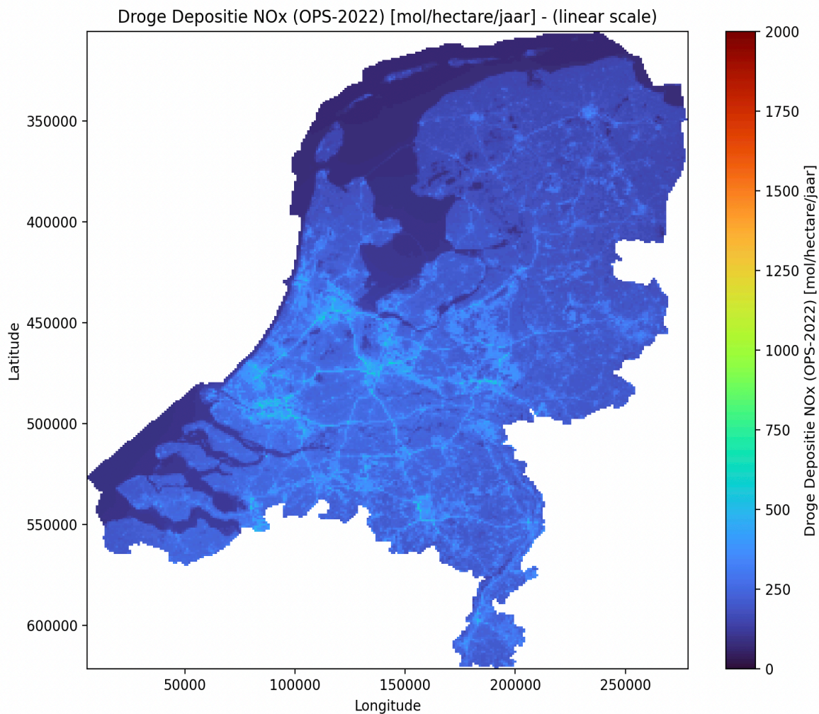
Figuur 9a: berekende droge NO x depositie per vierkante kilometer en uitgedrukt in mol per hectare per jaar. De dataset is gegenereerd met OPS 2022. De schaalverdeling is lineair en afgetoet op 2000 mol waardoor de kleuring van deze kaart identiek is aan de ammoniak-kaart (Figuur 7a). Wegverkeer geeft een duidelijke emissie, gevolgd door lokale depositie. Ook de steden (ruwheid) ervaren een iets hogere depositie aldus OPS 2022. Duidelijk is het effect – weinig verspreiding – van NO x te zien, ook hier zijn duidelijke gradiënten over het land gemodelleerd.
