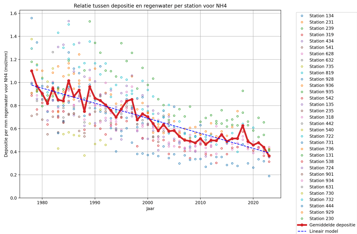
Figuur 6: De natte depositie data van alle stations is gedeeld door de werkelijke regenval op dat station in dat jaar om tot een depositie per millimeter regenwater te komen. Deze parameter kan gezien worden als een jaarlijkse concentratie term en daarmee een indicator voor 'de kwaliteit' van de lucht in dat jaar. De meeste pieken en dalen die sterk afwijken van het (arbitrair) gekozen lineaire model zijn te verklaren doordat er in het betreffende jaar sprake was van extreme droogte of juist natheid. We zien dat de ammoniak deken boven Nederland met ongeveer 60% is gedaald.
