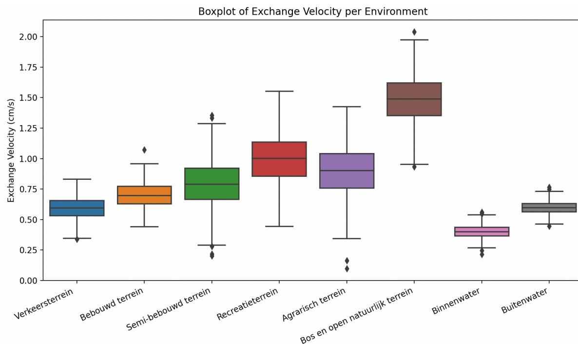
Figuur 9: Boxplot van de depositiesnelheid inschattingen op basis van de literatuur data. We hebben een normale verdeling verondersteld. Gemiddelde en standaarddeviatie staan in Tabel 9. Resultaat van de Monte Carlo simulatie N=500.
