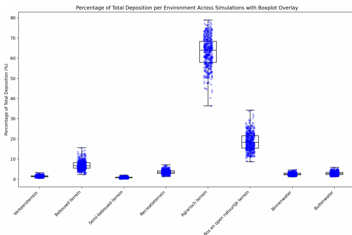
Figuur 14: Resultaat van een Monte Carlo simulatie N=500, waarbij de voorspellingen uitgedrukt zijn als percentage van de totale voorspelde droge depositie. De gemiddelde verdeling van ammoniakdepositie over de verschillende land categorieën staat ook in Figuur 14.
