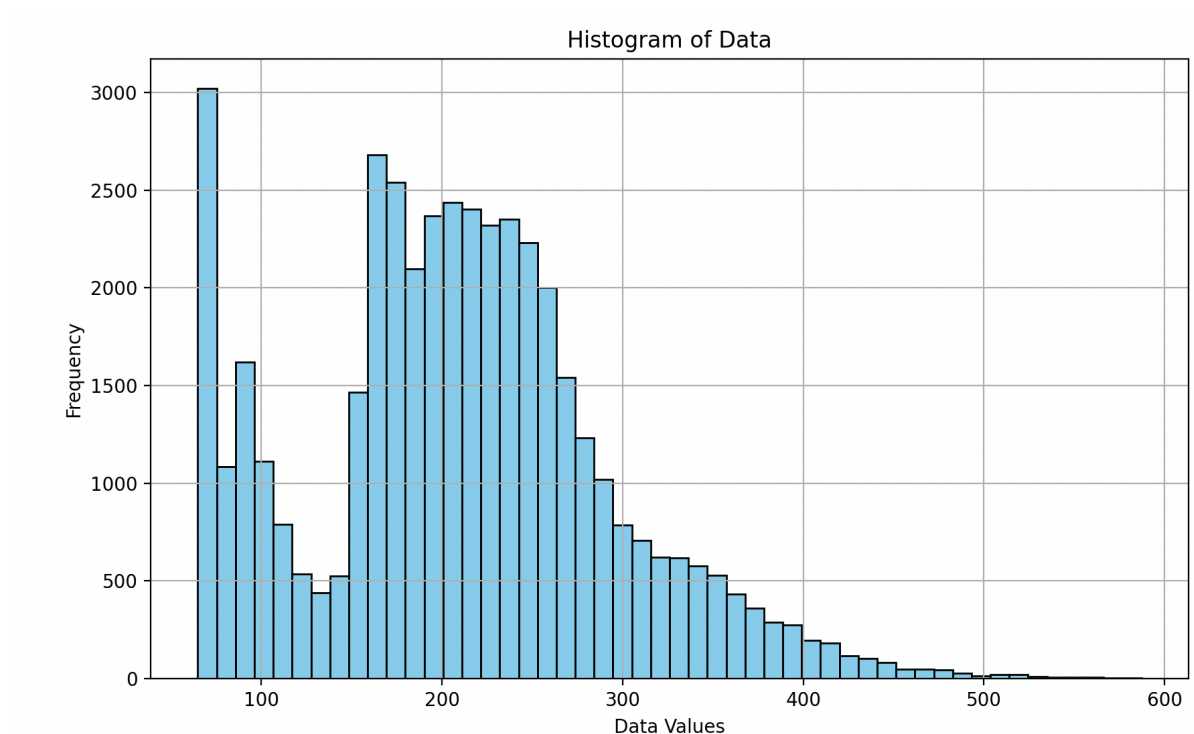
Figuur 10b: Histogram van droge NOx depositie in mol/hectare/jaar zoals berekend is door OPS 2022. De GDN kaart is opgedeeld in 43959 cellen van elk 1x1 km.
