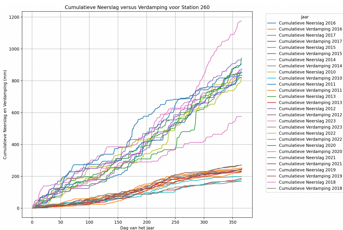
Figuur 11: Eerste analyse op De Bilt (station 260) gebruikt makend Penman-Monteith model en de werkelijk gemeten weerdata van het KNMI. Werkelijk gemeten neerslag en de berekende verdamping zijn uitgezet in deze grafiek voor de periode 2010 tot en met 2023.
