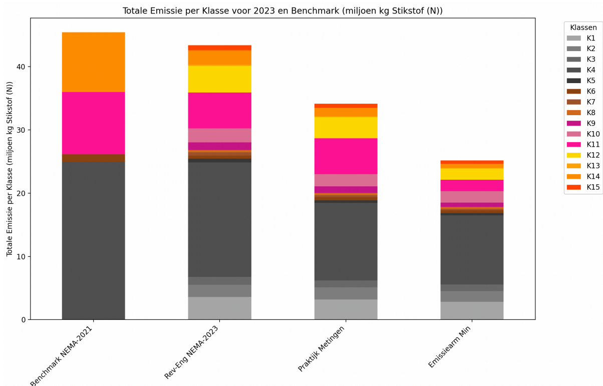
Figuur 7: Ammoniakemissie uitgedrukt in miljoen kilogram stikstof voor het jaar 2023.
