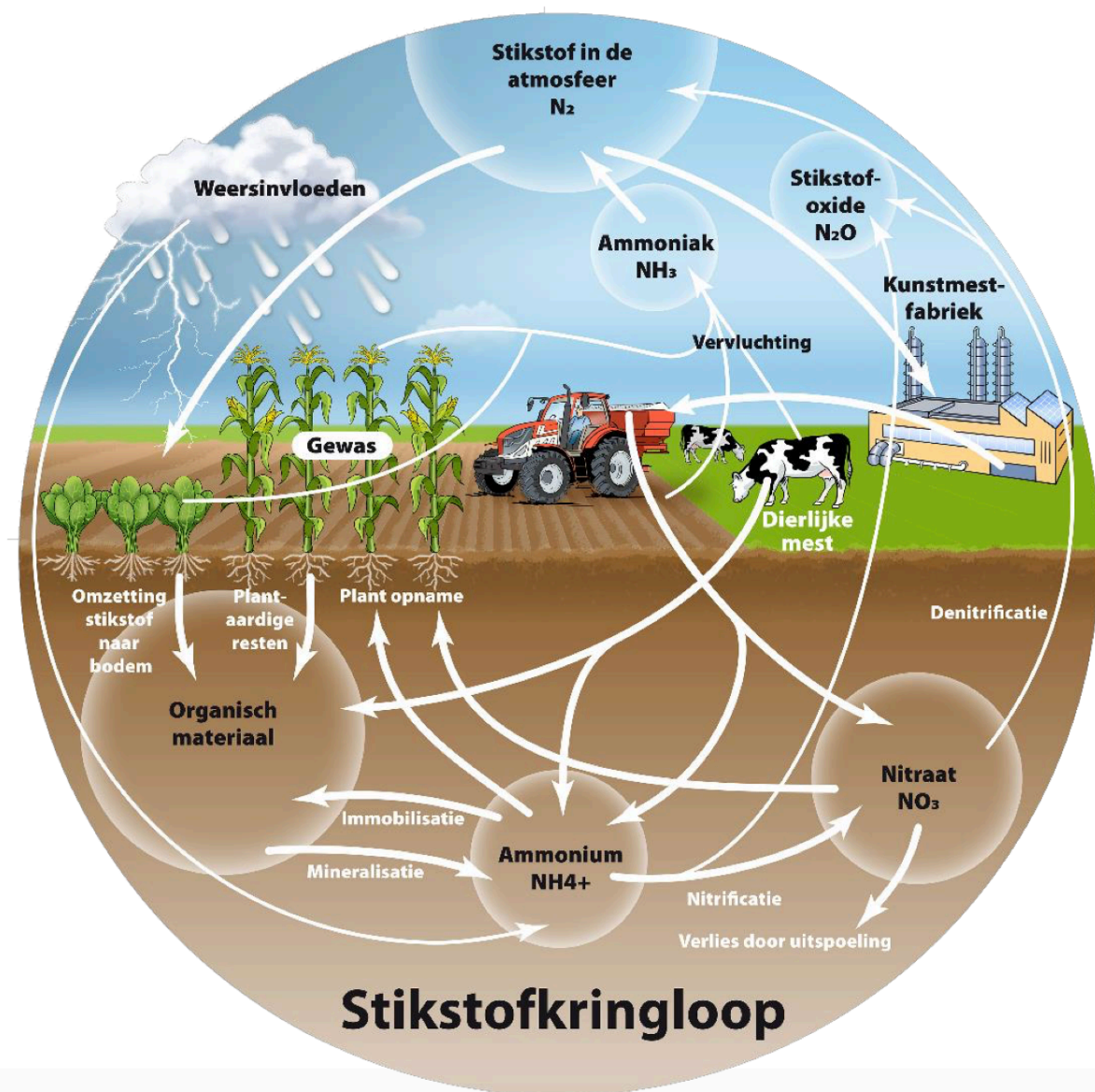
Figuur 2: De stikstofkringloop visueel uitgelegd met daarin de belangrijkste processen. Plaatje is overgenomen van een rapportage van de WUR).
