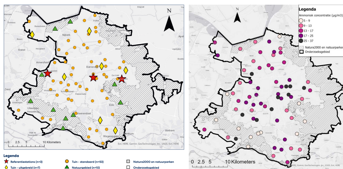
Figuur 12: lokaal meetnetwerk op initiatief van Regio FoodValley in de Gelderse Valley. Links de meetlocaties, rechts de gemiddelde concentratie ammoniak in de lucht in de periode maart tot en met augustus 2022. In de Natura 2000 gebieden bijvoorbeeld op de Utrechtse Heuvelrug zien we dat de concentratie rond de 5-9\mu\text{g}/\text{m}^3 is, terwijl 10 km verderop midden in het gebied met de hoogste concentratie aan dierhouderij de ammoniak concentratie volgens dit meetnetwerk bijna 40\mu\text{g}/\text{m}^3 is.
