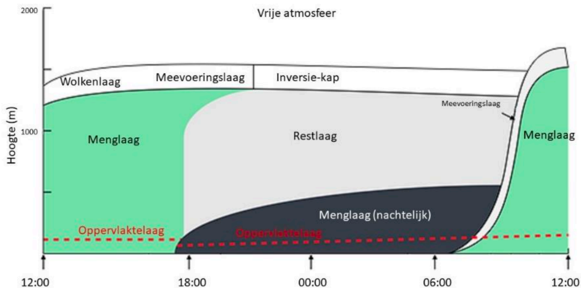
Figuur 2: Schematische weergave van de 24 uurscyclus van de atmosferische menglaag. 's Nachts is deze laag typisch tientallen tot enkele honderden meters hoog, gedurende de dag – afhankelijk van het weer – kan deze tot enkele kilometers hoog zijn. Bron: TNO-2024 en Stull, 1988.
