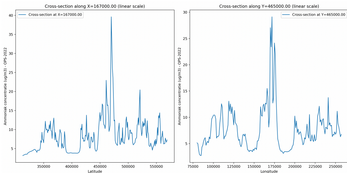
Figuur 6b: Horizontale en verticale doorsnede van bovenstaande heatmap met een resolutie van 1 kilometer. Links zien we de voorspelde ammoniak concentratie boven de Waddenzee, daarna de kop van Friesland, een stuk IJsselmeer, Flevoland en daarna de piek in de Gelderse Vallei. Rechts zien we Noord-Holland, de Utrechtse Heuvelrug en daarna de piek Gelderse Vallei, de lage plekken zijn de Veluwe en daarna verhoogde concentraties bij de Achterhoek
