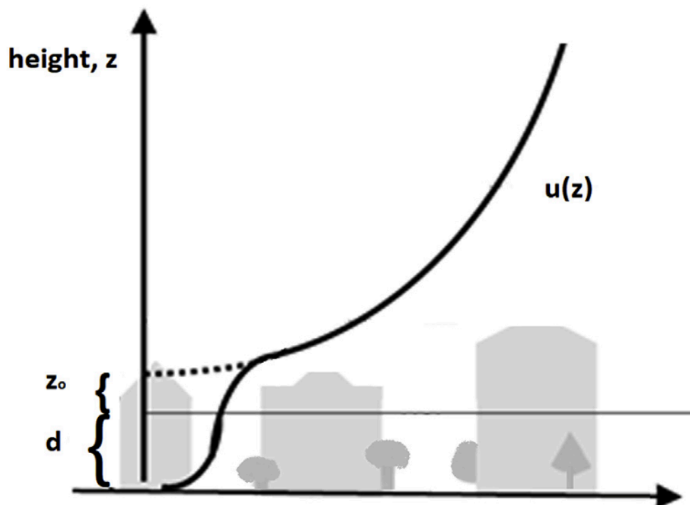
Figuur 1 – Windprofiel als functie van hoogte boven een ruw oppervlak aldus de theorie. z_0 is de ruwheidslengte en d wordt ‘zero plane displacement length’ genoemd. Het vertegenwoordigt een effectieve hoogte boven de werkelijke fysieke grond waarbij de windsnelheid theoretisch zou worden gereduceerd tot nul door de obstakels, zoals hoge vegetatie of gebouwen. Het verschuift effectief het nulpunt van de hoogtemetingen die worden gebruikt in het logaritmische windprofiel naar boven, wat de gemiddelde hoogte weerspiegelt waarop obstakels de luchtstroom blokkeren of verplaatsen. d wordt over het algemeen benaderd als ongeveer twee derde van de gemiddelde hoogte van de ruwheidselementen op het oppervlak (bijv. de bladerdakhoogte van een bos).
