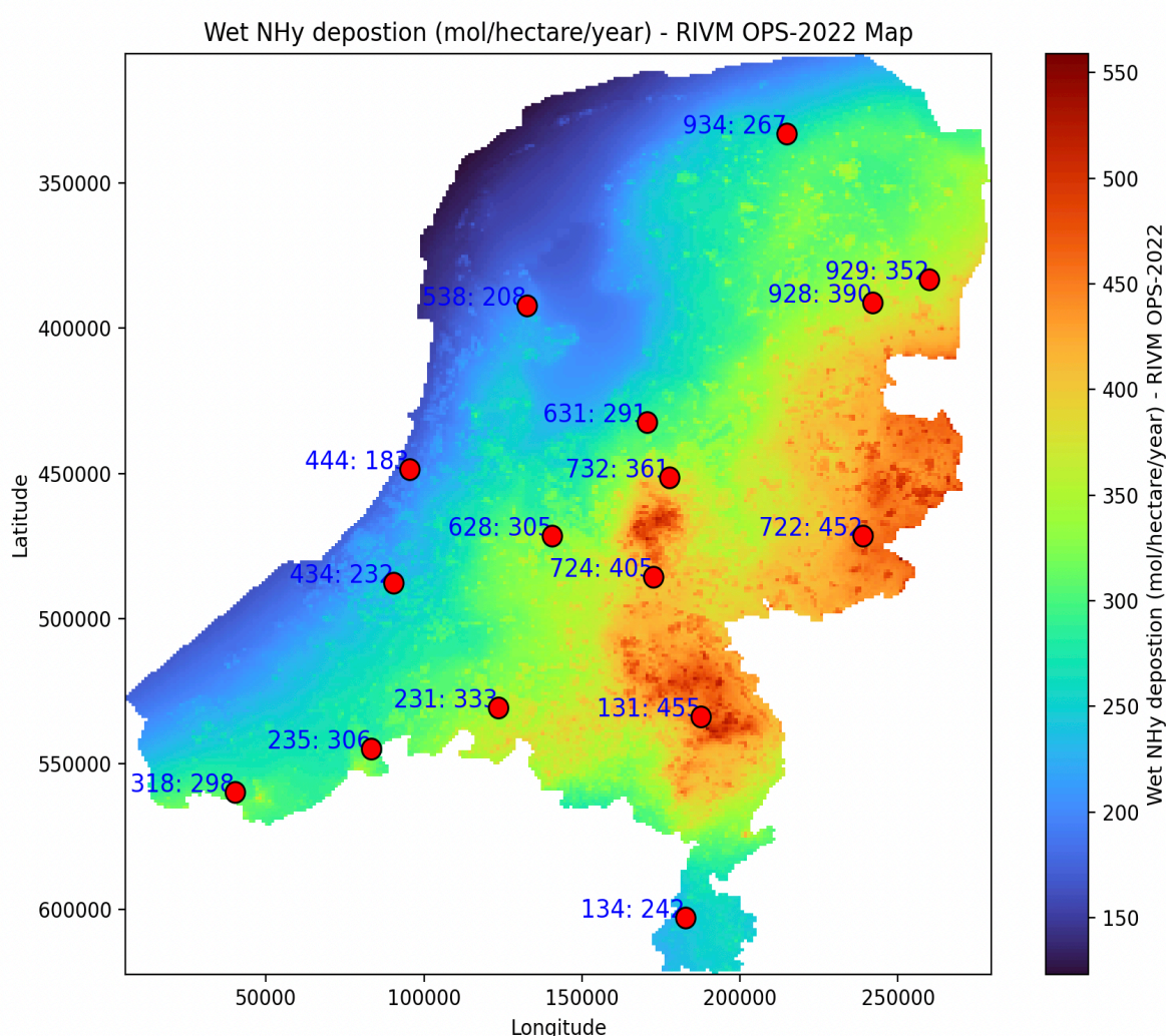
Figuur 3: de berekende natte ammoniak depositie boven Nederland (OPS-2022, data RIVM). Op de kaart staan met de rode stippen de regenmeetstations met achter het nummer de berekende natte depositie op die locatie. De berekende natte depositie is, zoals we verwachten lokaal op de Gelderse Vallei en de Peel hoog. Ook opvallend is de lage natte depositie aan de kust (en het Groene Hart) en de relatief hoge depositie in de Achterhoek.
