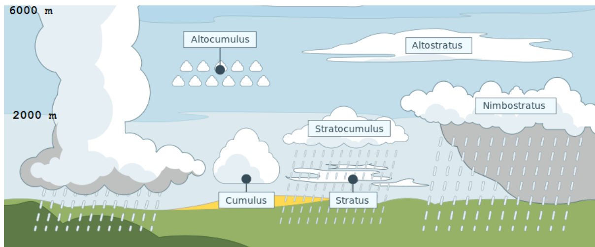
Figuur 3: Typische wolken boven Nederland. Wolken bevatten veel water waarin met name Ammoniak goed oplost. Wolken (met in regendruppels en in aerosol opgelost ammoniak) verplaatsen met een snelheid van ongeveer vijf tot dertig kilometer per uur vooral in het horizontale vlak. In Nederland is er een wind overwegend uit het zuid-westen waardoor mogelijk ammoniak vooral naar het oosten van Nederland en Duitsland getransporteerd kan worden.
