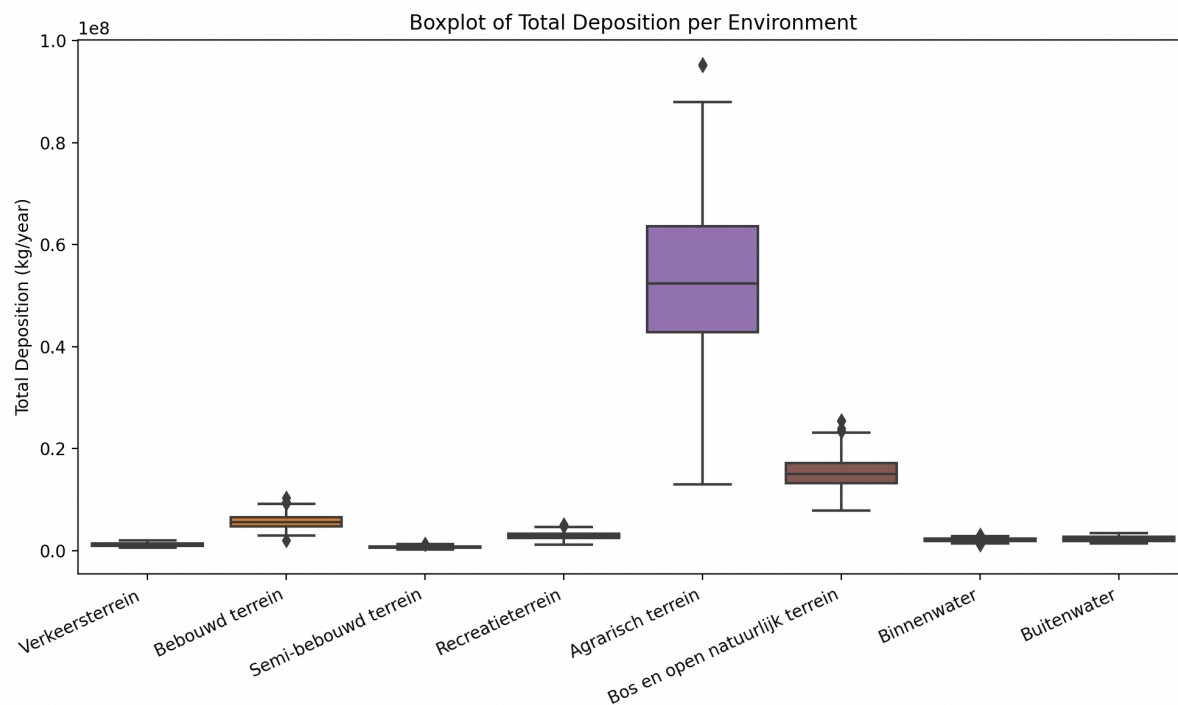
Figuur 13: Boxplot van de verwachte jaarlijkse depositie per landcategorie uitgedrukt in kilogram per jaar per gebied. De depositie op landbouwgebied is ongeveer 53 miljoen kilogram ammoniak, bos en natuur is 15 miljoen kilogram ammoniak en 5,5 miljoen kilogram ammoniak op bebouwd terrein. Resultaat van een Monte Carlo simulatie N=500.
