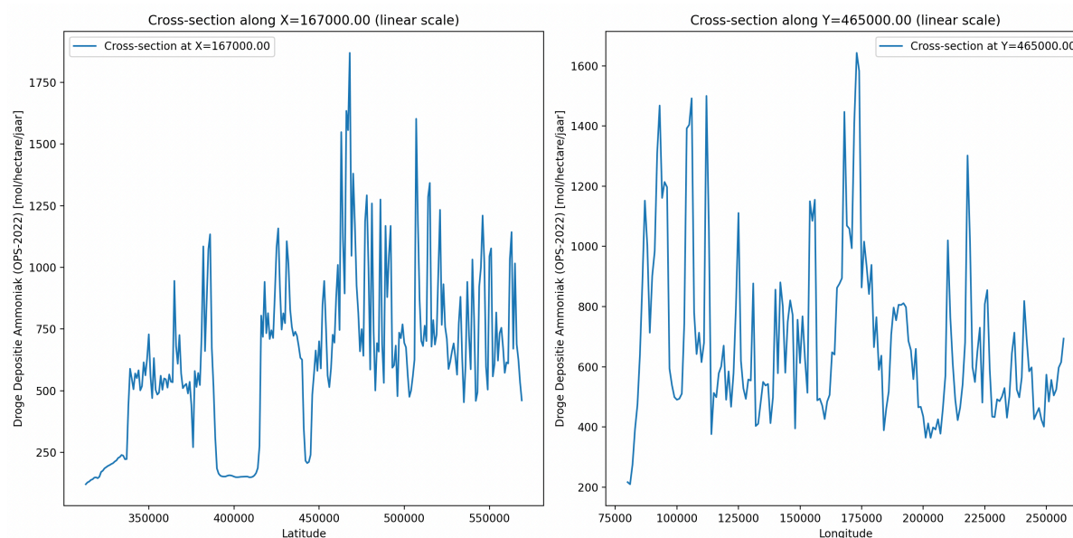
Figuur 8b: Doorsnede Noord-Zuid (links) en Oost-West (rechts). Let op! De schaal is niet hetzelfde.
