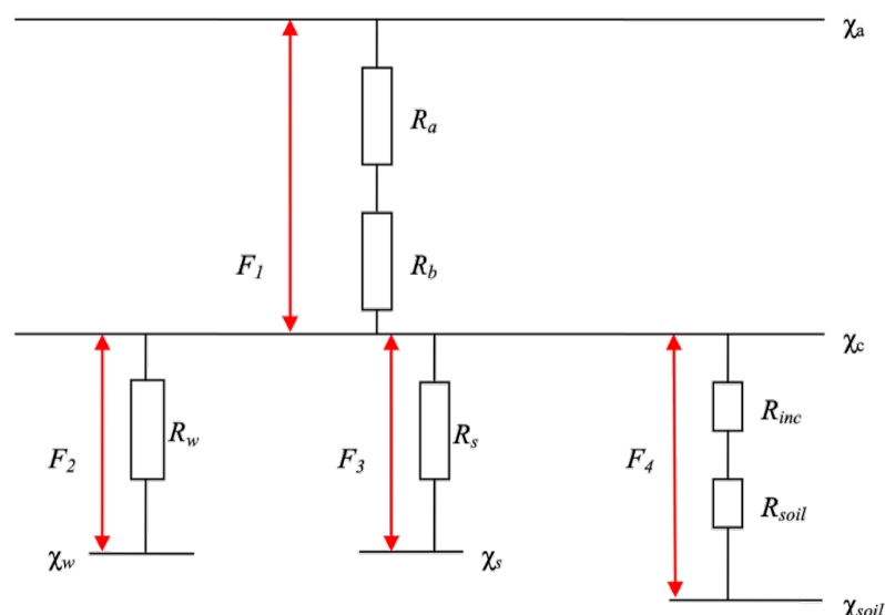
Figuur 5 – DEPAC-weerstandsmodel om droge depositie snelheid van ammoniak te bepalen R_a is de Aerodynamische weerstand, R_b is de Laminaire grenslaagweerstand en R_c (Oppervlakteweerstand ook wel Canopy Resistance genoemd). R_c is opgebouwd uit drie parallelle weerstanden in DEPAC. Bron: RIVM.
