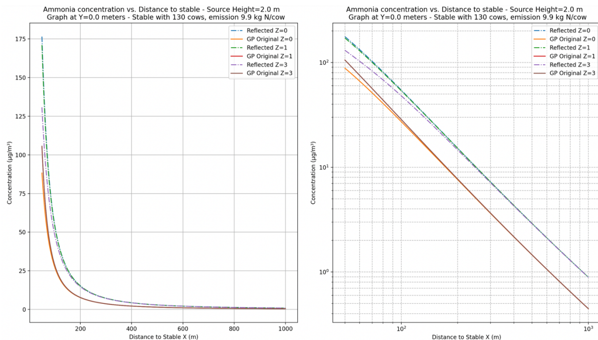
Figuur 17b – Berekende ammoniakconcentratie met een eenvoudig Gaussian Plume model (met reflectie, maar zonder depositie) uitgedrukt in \mu\text{g}/\text{m}^3 ten opzichte van de afstand van een stal uitgedrukt in meters. De berekende concentratie komt redelijk overeen met de gemeten literatuurdatta uit figuur 15a.
