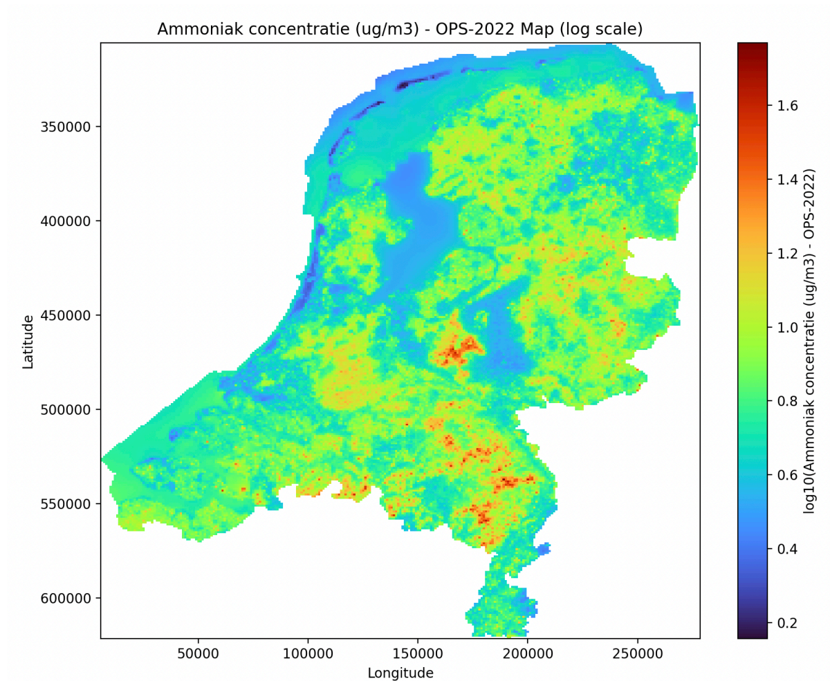
Figuur 7: Concentratie heatmap (OPS-2022) van de ammoniak concentratie uitgedrukt in \mu\text{g}/\text{m}^3 op een 1 \times 1 \text{ km} grid over Nederland op een logaritmische schaal. Deze visualisatie benadrukt die locaties waar ammoniakemissies – vooral vanuit stallen – hoog zijn. Deze kaart illustreert tevens de lokaliteit van het stikstof problemen goed. Ammoniak is vooral een lokaal milieu-onderwerp.
