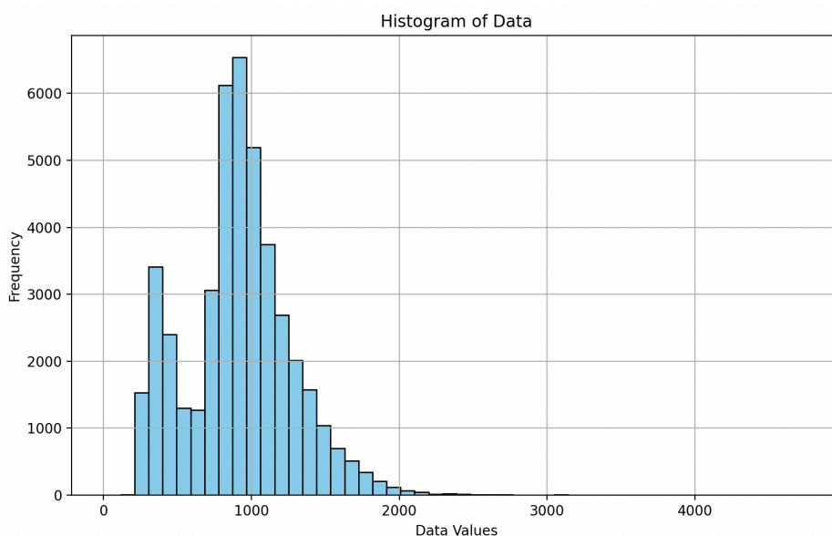
Figuur 8: Histogram van de berekende totale ammoniak depositie (nat en droog) boven Nederland uitgedrukt in mol stikstof per hectare per jaar volgens de OPS-2022 berekening en op een 1km x 1km grid. Bron: databestand verkregen via RIVM zomer 2024.
