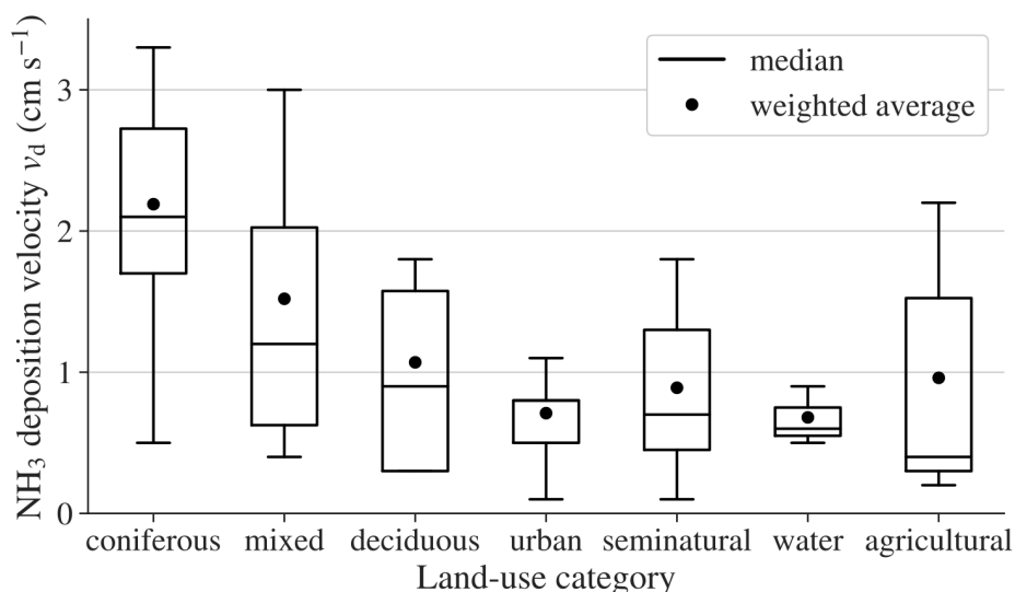
Figuur 7: Samenvatting van de depositiesnelheden uitgedrukt in centimeter per seconde. Figuur is overgenomen van het werk van Schrader (waaronder zijn proefschrift en artikel uit 2014). Deze grafiek is gebruikt om de tweede kolom in Tabel 4a te construeren.
