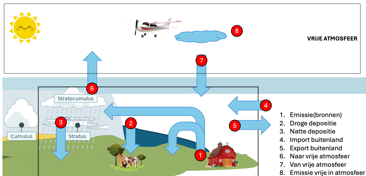
Figuur 5: Nederland weergegeven als een 'zwarte' doos. Ammoniak emitteert naar de lucht, en komt weer in de vorm van natte en droge depositie op de grond. Ammoniak kan ook via import uit het buitenland komen of via export naar het buitenland gaan. Tenslotte kan ammoniak naar hogere atmosfeer lagen gaan en/of afgebroken worden. De nummers in deze figuur corresponderen met de nummers in Tabel 1.
