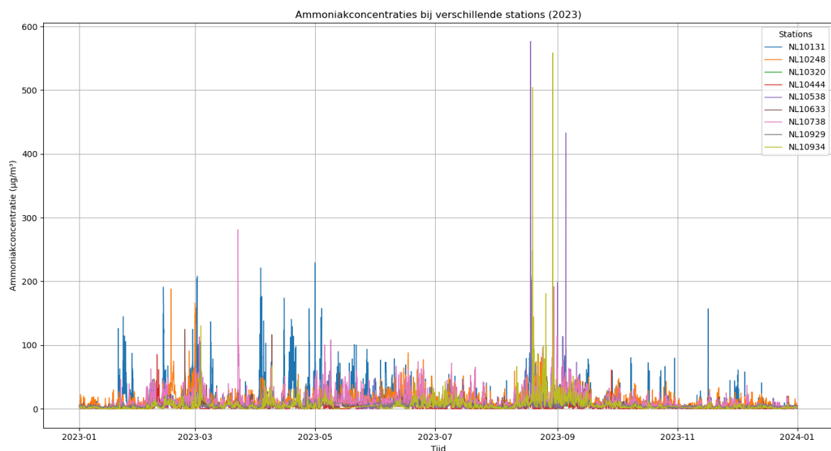
Figuur 8: Uur-metingen vanuit het LML netwerk (9 stations verspreid over Nederland. Ondanks dat de gemiddelde concentratie rond de 6 µg/m 3 is, zien we hier duidelijk de enorme pieken die soms gemeten worden. Waarden van 100 µg/m 3 worden normaal alleen gemeten in stallen. Voorzichtigheid is geboden om lukraak een gemiddelde concentratie waarde te bepalen op basis van deze LML metingen.
