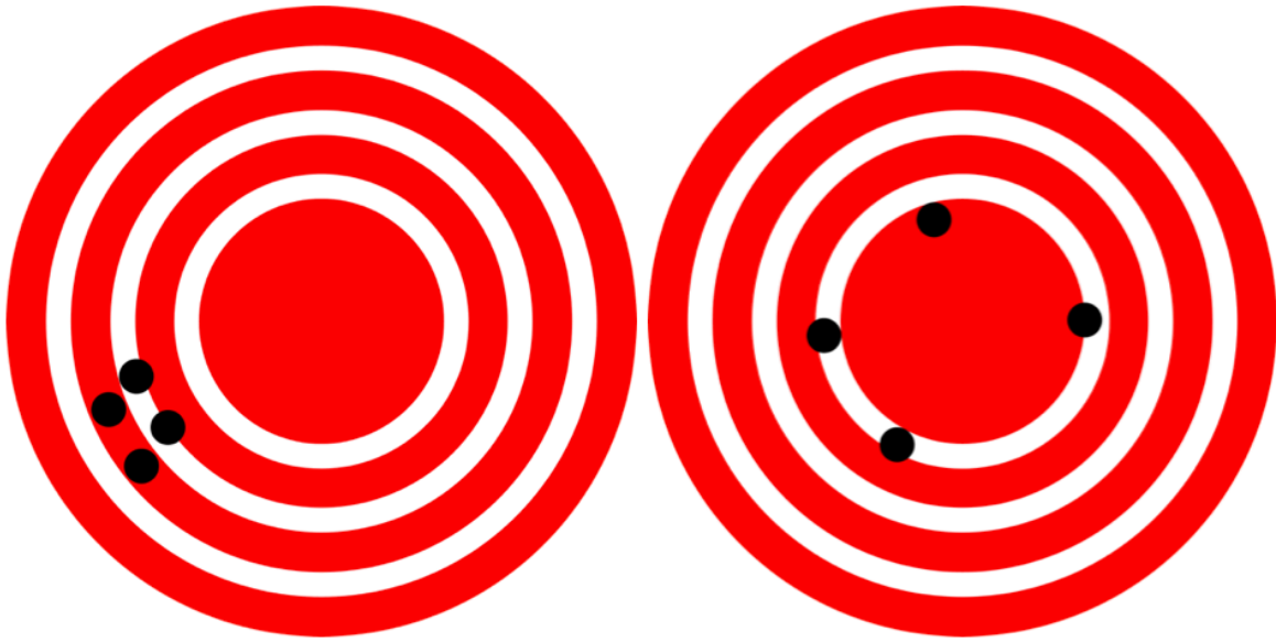
Figuur 3: In het linker plaatje zie je dat de precisie hoog is omdat de punten dicht bij elkaar liggen. Tegelijk zie je dat de juistheid laag is omdat ze ver van de roos af zitten. Dat duidt op een systematische fout. In het rechter plaatje zie je dat de juistheid beter is, maar de precisie lager. In dat geval zit er minder afwijking in het instrument dat we gebruiken om de werkelijkheid vast te leggen in een waarde.
