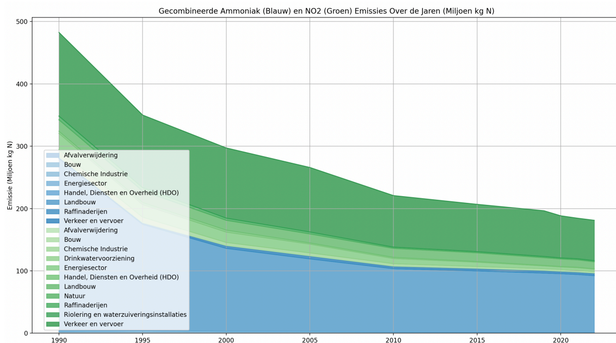
Figuur 1: Verloop van de stikstof emissie sinds 1990. De blauwe tinten gaan over ammoniak, en de groene tinten over NO x . Op de y-as staat "miljoen kilogram stikstof" waardoor de vergelijking correct is. Vooral de enorme afname van de hoeveelheid ammoniak uitstoot is opvallend. Deze getallen komen uit modellen, vooral het NEMA-model wordt voor de landbouw emissies ingezet.
