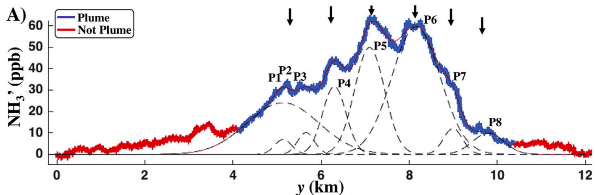
Figuur 13: Uit Leifer et.al. (2018) Acht-pluim geïnformeerd (8I) model voor I-15 downwind (noord naar zuid) transect met betrekking tot willekeurige laterale afstand ( y ) voor A) ammoniak anomalie ( \text{NH}_3 ) en winden ( u ) versus ( y ). Pluimpieken zijn gelabeld. Pijlen tonen gemodelleerde kenmerken die een model met zes pluimen suggereerden.
