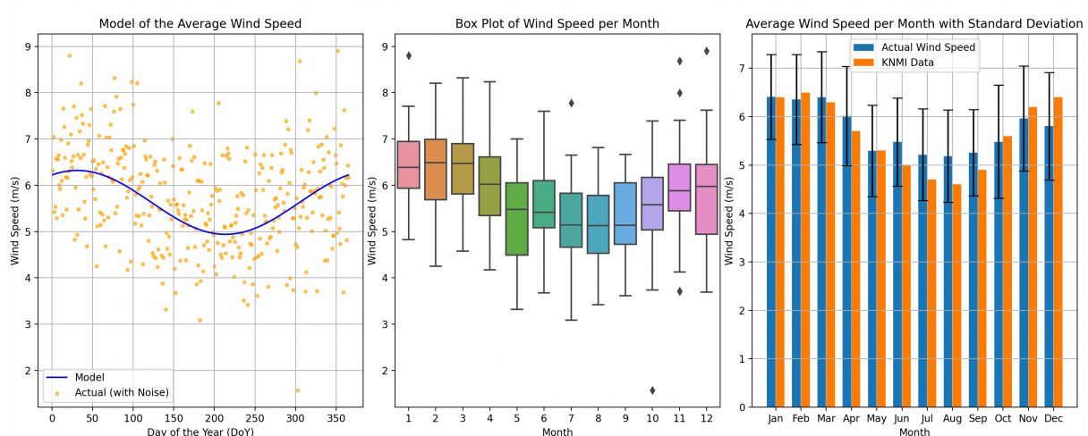
Figuur 3a – Windmodel met randomizer voor Nederland (links en midden). Dit model wordt gebruikt om de variatie van de windsnelheid op de R_a en R_b waarden te onderzoeken. Gemiddelde gemeten windsnelheid (KNMI) is weergegeven rechts.
