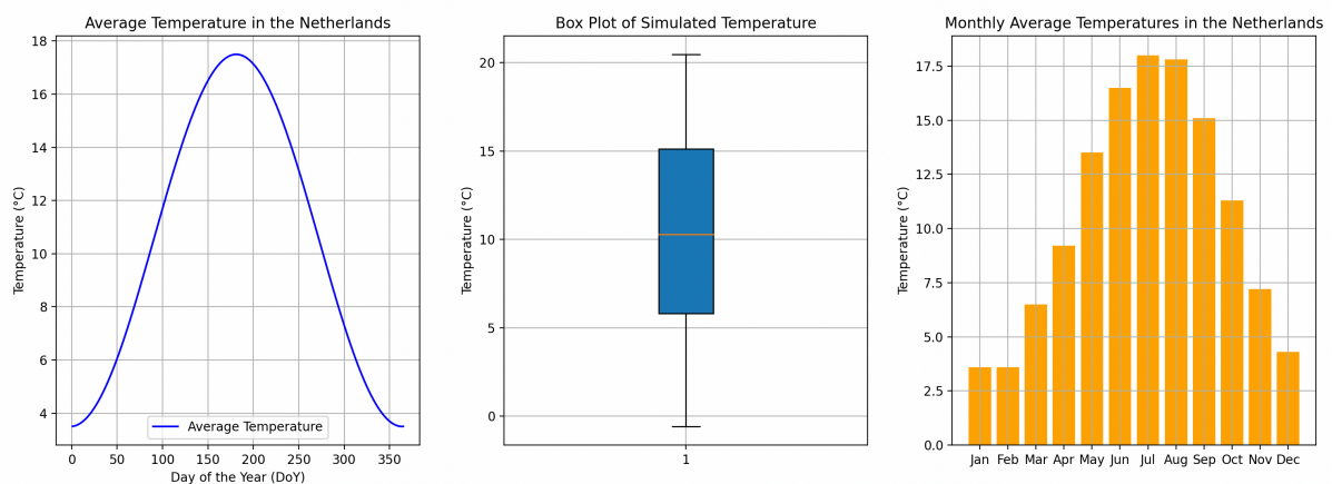
Figuur 3b – Temperatuurmodel zonder randomizer voor Nederland (links en midden). Dit model wordt gebruikt om de variatie van gemiddelde temperatuur in Nederland op verschillende parameters in het model te bepalen. Gemiddelde gemeten maand-temperatuur (KNMI) is rechts weergegeven.
