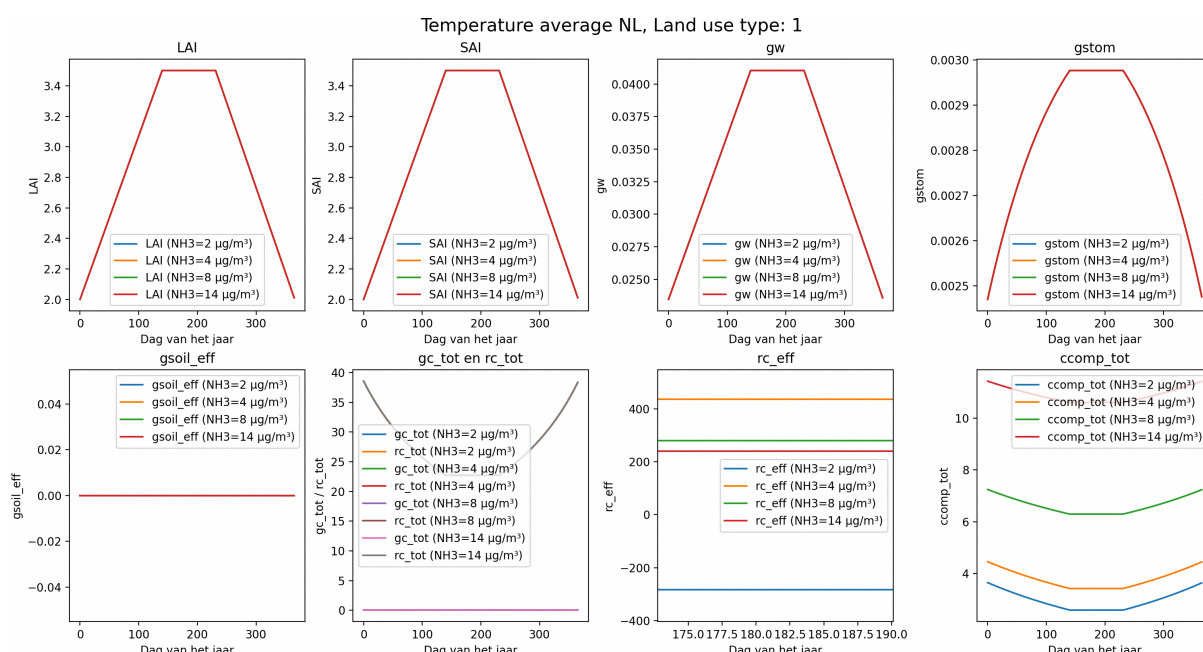
Figuur 6a – DEPAC (Vanuit Fortran90 omgezet naar Python, validatie van de code heeft niet plaatsgevonden), land-type 1 (grasland). Jaargemiddelde R_c zit tussen de 40 en 23 sec/m. Compensatiepunt ( C_{comp\_tot} ) is afhankelijk van de ammoniakconcentratie ( c_{atm} ) buiten, bij een typische c_{atm} van rond de 8 \mu\text{g}/\text{m}^3 ligt C_{comp\_tot} rond de 6 \mu\text{g}/\text{m}^3 . Disclaimer: DEPAC_Python is niet gevalideerd.
