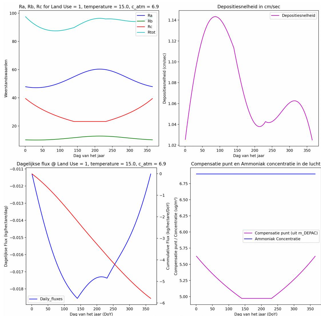
Figuur 7: output of DEPAC_Python module. Linksboven de berekende R_a , R_b en R_c waarde, rechtsboven de depositiesnelheid in cm/sec, linksonder de flux per dag (blauw) en de cumulatieve flux over alle dagen (DoY). Rechtsonder tenslotte het compensatiepunt (paars) en de ingestelde ammoniakconcentratie (blauw).
