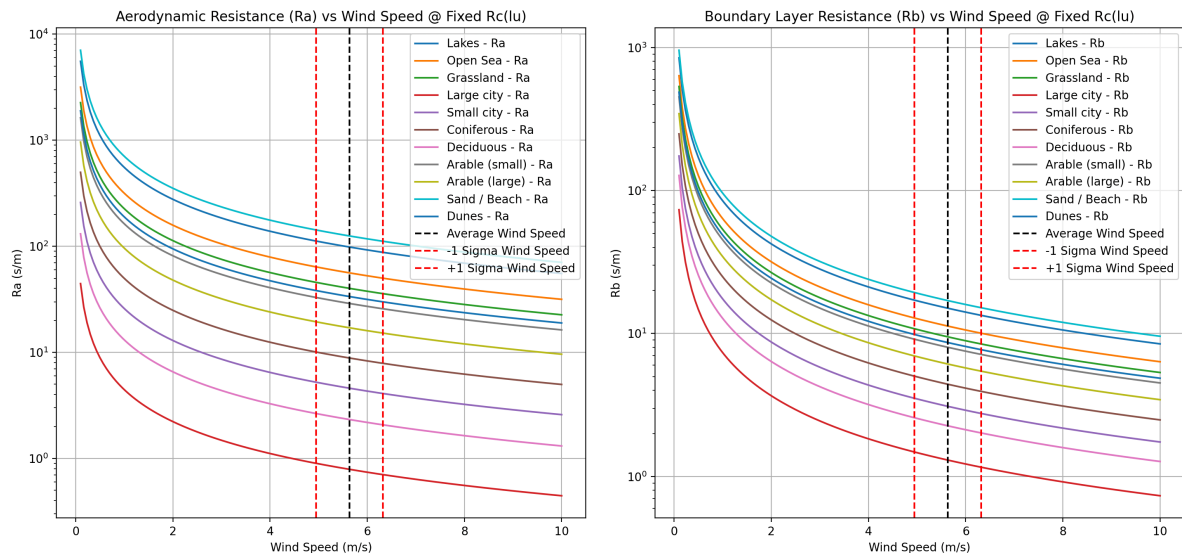
Figuur 4 – Effect van de windsnelheid op R_a (links) en R_b (rechts) bij de verschillende landtypen met elk een eigen ruwheden z_0 . De zwarte verticale stippellijn is de gemiddelde windsnelheid boven Nederland, de twee rode verticale stippellijnen geven de standaarddeviatie aan van de gemiddelde windsnelheid. Uit beide grafieken is duidelijk ook te concluderen dat de weerstand fors hoger wordt bij een lage windsnelheid. Bij windstilte wordt er vrijwel geen nieuwe ‘ammoniak’ aangevoerd naar het oppervlak.
