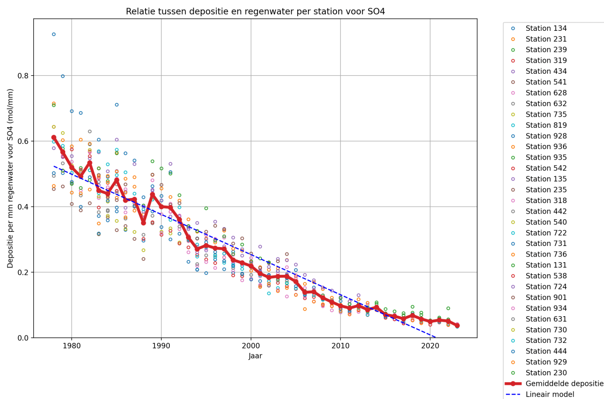
Figuur 9: Ondanks dat dit rapport vooral gaat over ammoniak en een beetje over stikstofoxiden is ter illustratie van praktisch milieubeleid – ontzwaveling van brandstoffen- deze grafiek van zwaveloxide geplot. Door juist emissiebeleid is de totale natte depositie met 90% gedaald in de betreffende periode. Ook bij deze chemische contaminant zien we de natte en droge jaren terug in de grafiek.
