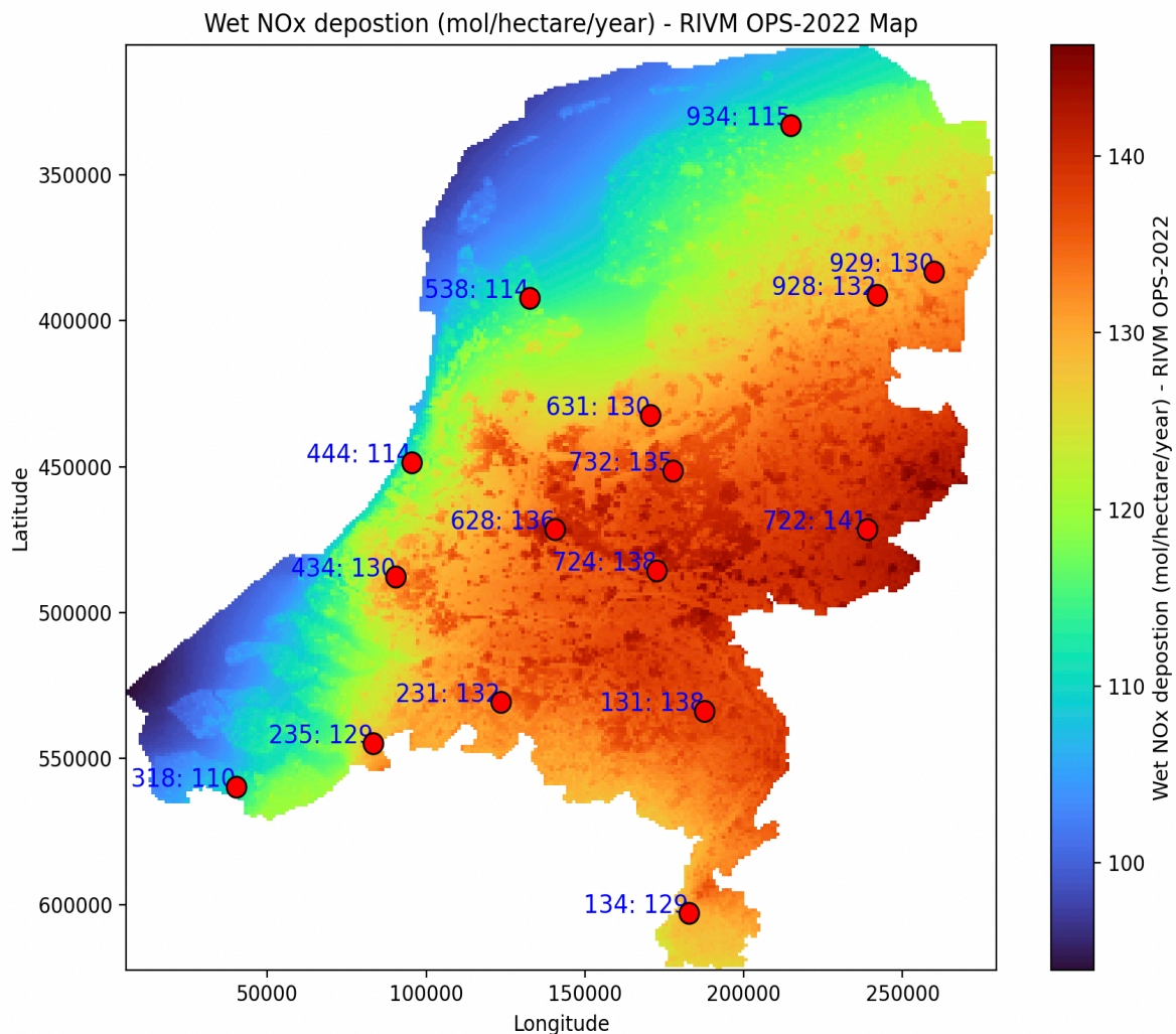
Figuur 4: de berekende natte stikstofdioxide (NOx) depositie boven Nederland (OPS-2022, data RIVM). Op de kaart staan - met de rode stippen aangegeven- de regenmeetstations met daarachter het station nummer en de berekende natte depositie op die locatie. Opvallend is dat de natte NOx depositie in het oosten van het land hoger is dan in het westen van het land. Dit terwijl de meeste emissies van NOx vooral in Noord en Zuid-Holland en Utrecht plaatsvinden. Het effect van de overwegend westelijke wind is waarschijnlijk de verklaring voor dit fenomeen dat wel nader onderzocht zou moeten gaan worden.
