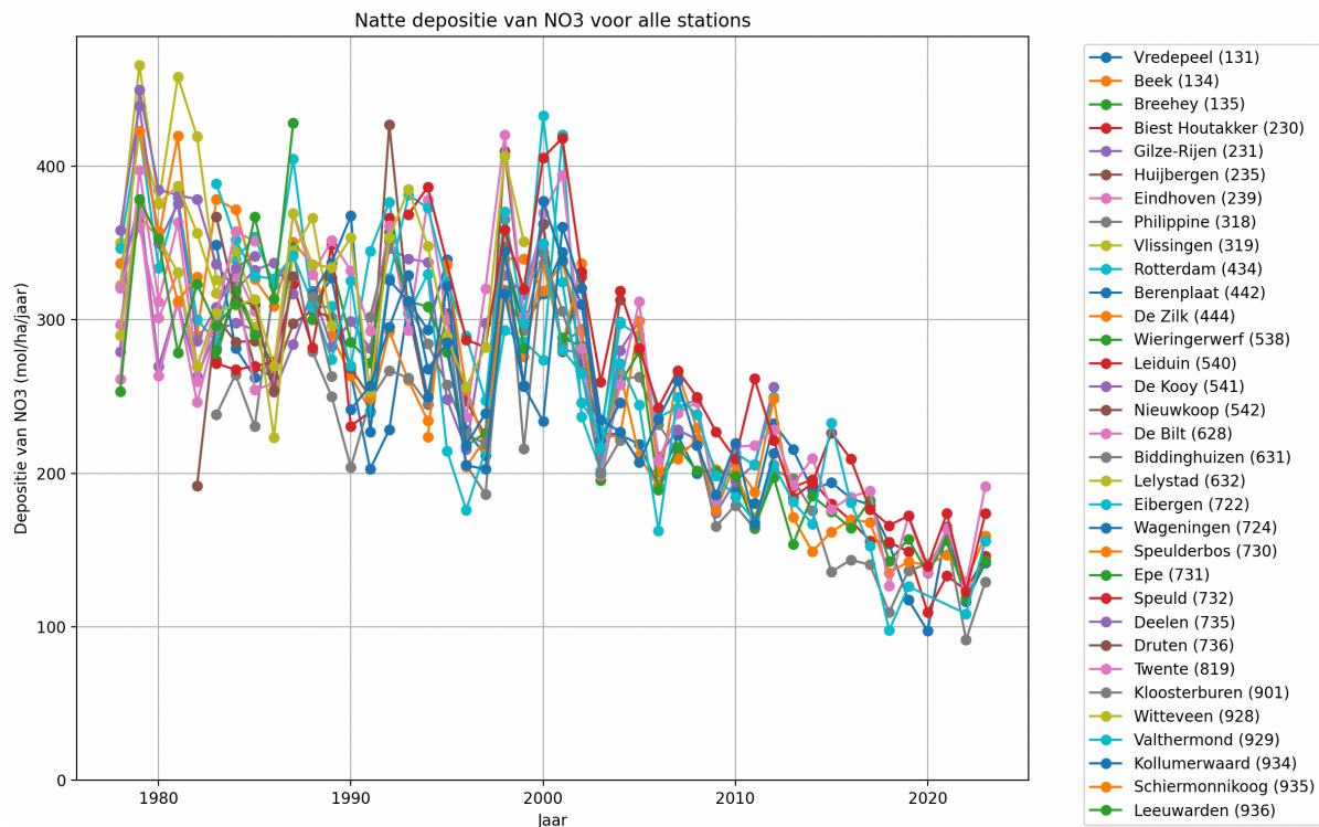
Figuur 2: alle beschikbare gemeten natte stikstofoxide depositiedata in Nederland vanaf 1978. Vanaf 2014 is het aantal meetpunten verder afgenomen. Volgens de metingen is de natte depositie op Nederland tussen de 100 en 175 mol per hectare per jaar.
