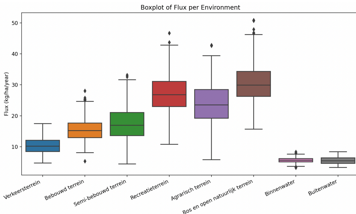
Figuur 13: Boxplot van de berekende droge depositie in kilogram ammoniak per hectare per jaar. De depositie is berekend door de ammoniak concentratie te vermenigvuldigen met de depositie-snelheid. Resultaat van de Monte Carlo simulatie N=500. De toelichting op deze berekeningen staat in het hoofdstuk “H4 Verspreiding en Massabalans over Nederland”.
