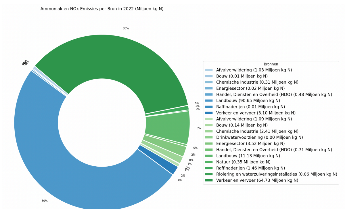
Figuur 2: Donut diagram met percentages voor het jaar 2022. De blauwe tinten gaan over ammoniak, en de groene tinten over NOx. Let op dat de sectoren tweemaal voorkomen in deze grafiek, eenmaal bij ammoniak en eenmaal bij NOx. Voor landbouw betekent het dat we 50% en 6% moeten optellen, totaal stikstof voor landbouw is 56% (zie ook Figuur 3). Getallen komen uit modellen.
