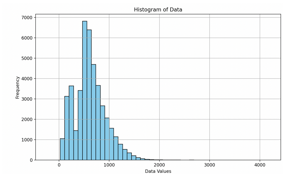
Figuur 10a: Histogram van droge ammoniak depositie in mol/hectare/jaar zoals berekend is door OPS 2022. De GDN kaart is opgedeeld in 43959 cellen van elk 1x1 km.
