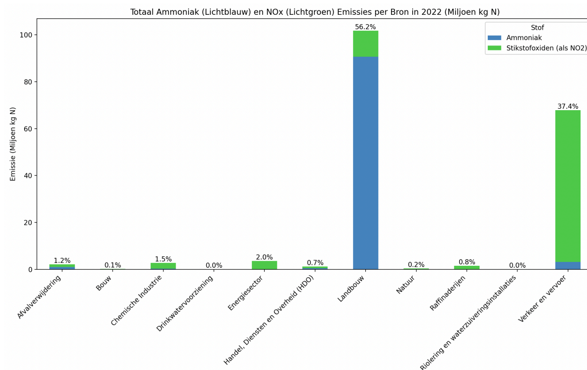
Figuur 3: Emissie naar de lucht per bron (2022) volgens de officiële emissie-registraties. Verkeer en vervoer en landbouw (vooral de dierhouderij) zijn de absoluut grootste emissie-bronnen naar de lucht in Nederland. De emissies van deze twee bronnen zijn echter berekend met modellen.
