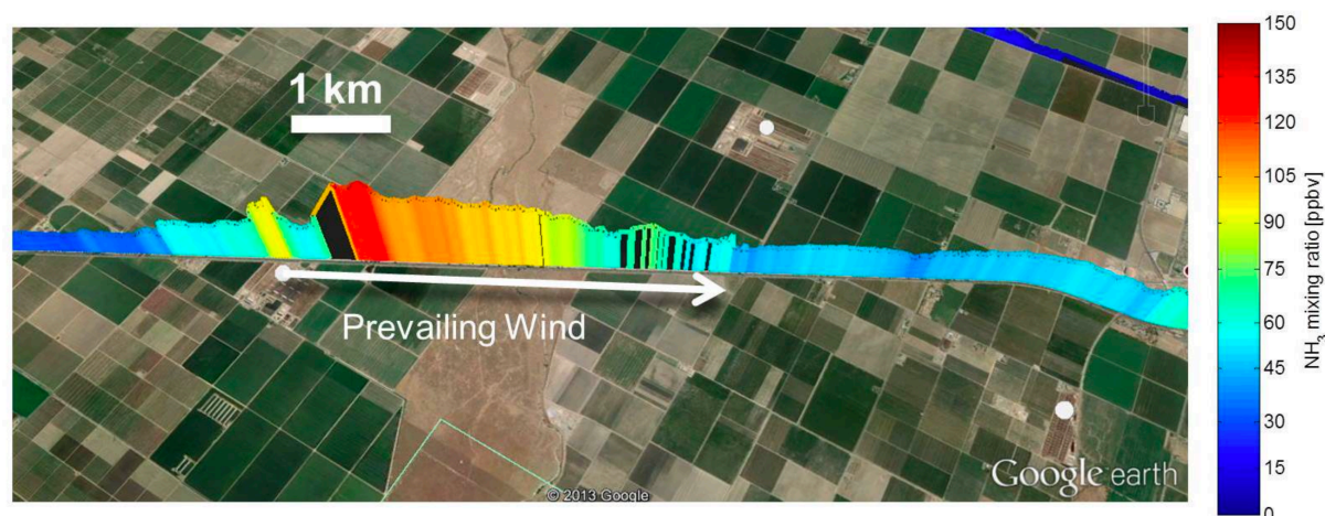
Figuur 16: Miller et.al. (2015), mobiele ammoniak concentratie metingen benedenwinds vanaf een feedlot. Feedlots zijn door hun massaliteit niet vergelijkbaar met de melkveehouderij in Nederland. Wel geven deze metingen een goede illustratie van de snelle verdunning van ammoniak op afstand vanaf een stal.
