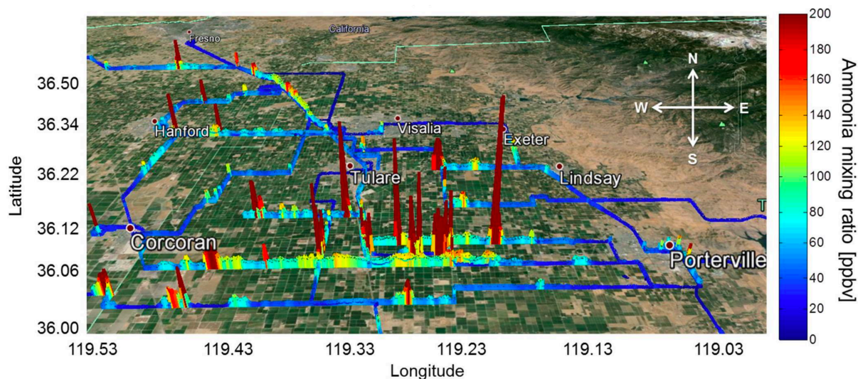
Figuur 15: Miller et.al. (2015), mobiele ammoniak concentratie metingen benedenwinds vanaf een feedlot. Feedlots zijn door hun massaliteit niet vergelijkbaar met de melkveehouderij in Nederland. Wel geven deze metingen een goede illustratie van de snelle verdunning van ammoniak op afstand vanaf een stal en daarmee de grote ammoniak gradiënten die we ook zien op de GCN van RIVM (Figuur 6b)
