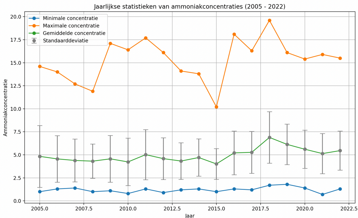
Figuur 3: Gemiddelde MAN ammoniakconcentratie per jaar inclusief de standaarddeviatie (jaargemiddeld en over alle locaties) om de spreiding over het netwerk te illustreren. De minimale en maximale concentraties zijn separaat weergegeven. De gemiddelde ammoniakconcentratie boven het MAN netwerk is 5,1 \mu\text{g}/\text{m}^3 en dat is ongeveer 0,7 \mu\text{g}/\text{m}^3 lager dan 'gemiddeld in Nederland'. Duidelijk is te zien dat het concentratie verloop over de afgelopen tien jaar constant is met kleine piekjes omhoog en omlaag. Opvallend is de piek in 2018 waarbij duidelijk de concentratie wat hoger is dan de voorgaande jaren. De maximale concentraties worden gemeten op de Bennekomse Meent (oranje lijn), en de laagste concentraties worden op Meyendel, Vlieland, Zwanenwater, Terschelling gemeten.
