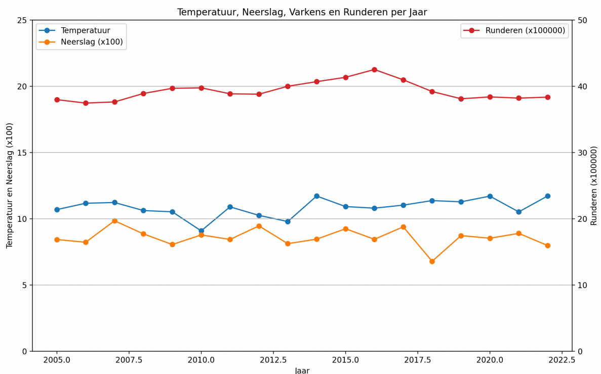
Figuur 4: CBS en KNMI-gegevens versus jaar. Voor de leesbaarheid van de grafiek is het aantal runderen gedeeld door 100.000 (secundaire y-as) en is de regenval gedeeld door 100 (primaire y-as). Opvallend is het droge jaar 2018 en de piek in het aantal runderen in 2016 gevolgd door een snelle afname in de jaren 2017 en 2018 als gevolg van een verplichte reductie.
