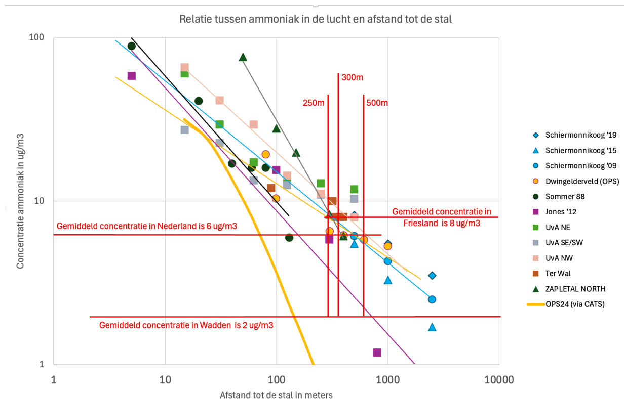
Figuur 17a – Gemeten ammoniak concentratie uitgedrukt in \mu\text{g}/\text{m}^3 ten opzichte van de afstand van een stal uitgedrukt in meters. De drie horizontale lijnen geven aan wat de verschillende achtergrond concentraties zijn van de stikstofdeken op grotere afstand.
