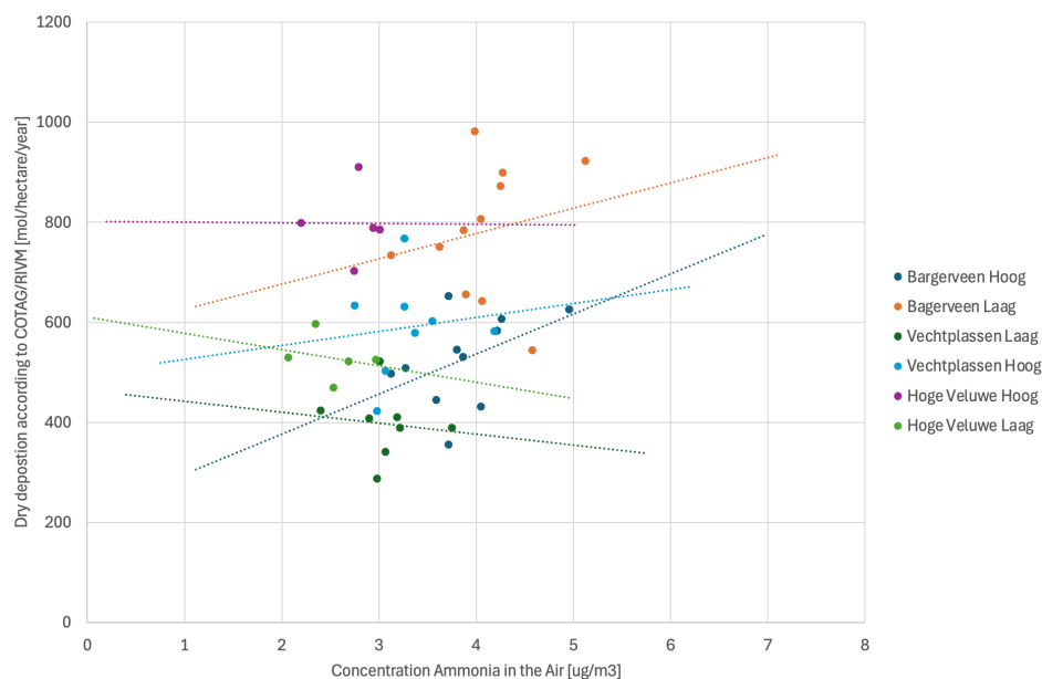
Figuur 6 : resultaat van de droge depositie 'metingen' via COTAG. COTAG meet de concentratie en via een berekening wordt de flux (depositie) geschat. Er staan drie COTAG palen in Nederland. Deze grafiek geeft de gemeten concentratie vs. de gemodelleerde COTAG droge depositie weer. Bron: RIVM Website.
