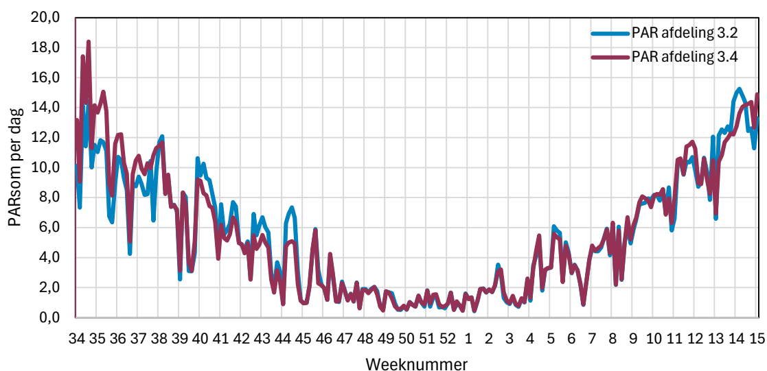
Figuur 7: Gerealiseerde PAR-sommen in afdelingen 3.2 en 3.4. Gemeten met priva par-sensoren in het midden van de kas
