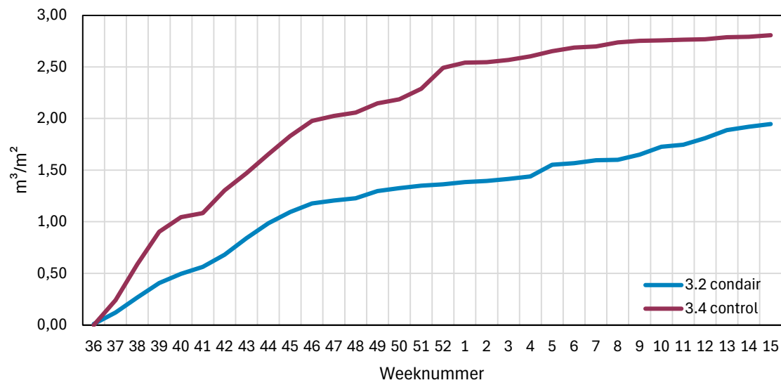
Figuur 13: gasverbruik in m³ per m² in afdeling 3.2 en 3.4 (control)
