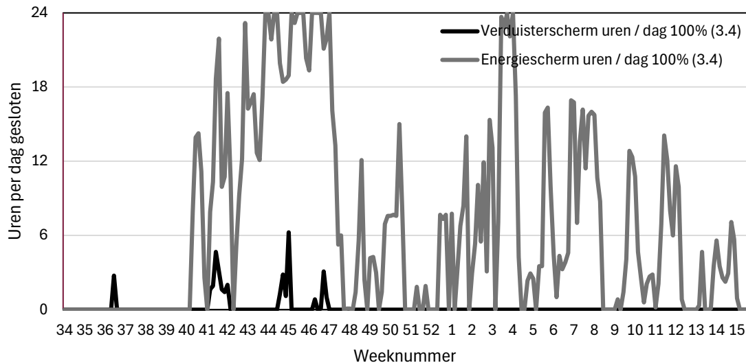
Figuur 11: Sluiting energie- en verduisterschermbloot op 100% in uren per dag in afdeling 3.4 (control)
