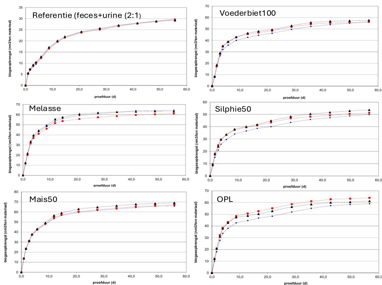
Figuur 4-9 De ontwikkeling van de biogasopbrengst over een periode van 56 dagen in Nm 3 per ton gemeten door Opure. Voederbiet100 is 100 g ds voederbiet per 2 kg mest, Mais50 en Silphie50 = 50 g ds mais of silphie per 2 kg mest elk met 3,5% melasse, OPL is 18%OPL toevoeging, melasse is 5,1% melasse toevoeging. Behandelingen met mais, voederbieten en silphie werden vooraf aangezuurd tot een pH van 6,2 met azijnzuur.
